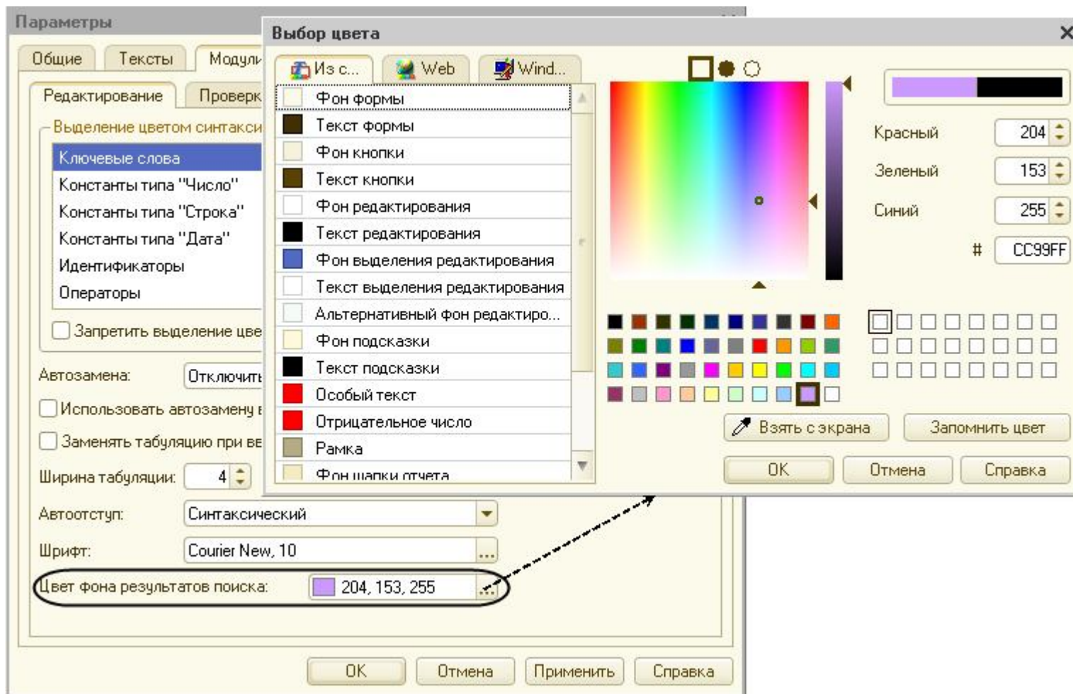
Рис. 46. Настройка подсветки результатов поиска
