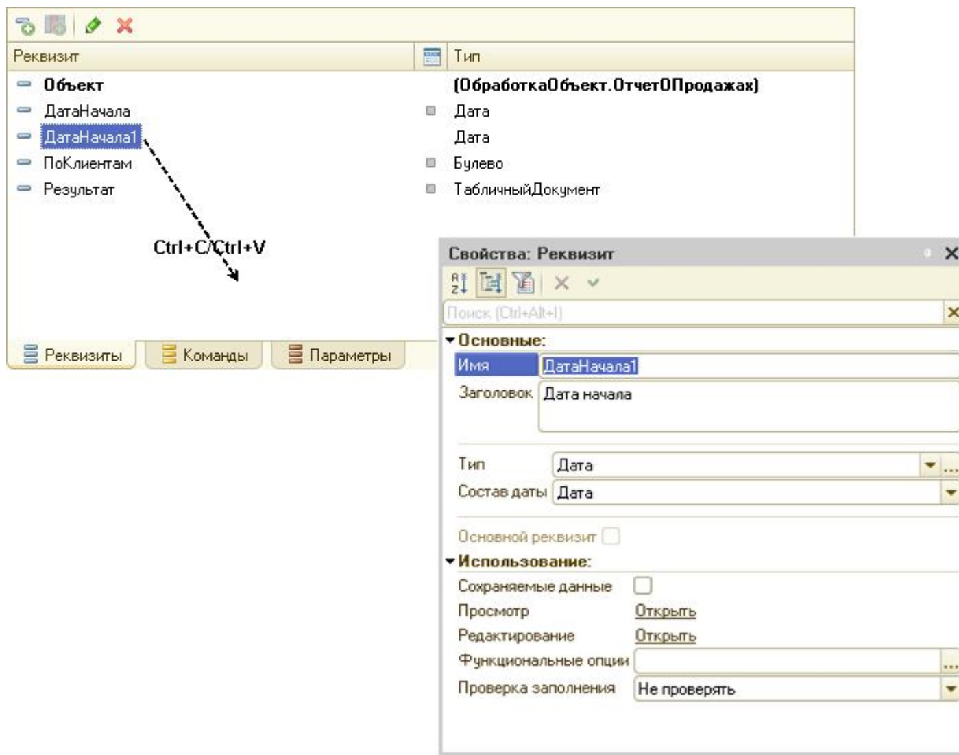
Рис. 77. Копирование реквизитов в редакторе формы
