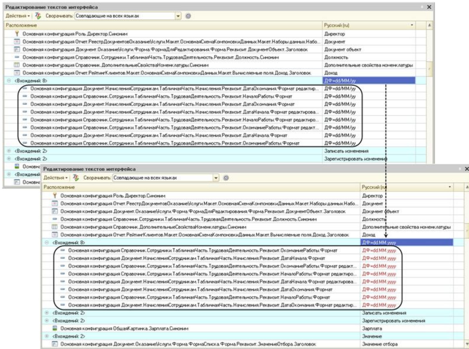
Рис. 183. Редактирование текстов интерфейса
