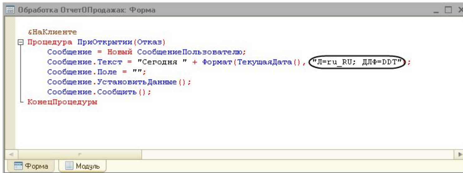
Рис. 130. Текст процедуры «ПриОткрытии» в модуле формы
