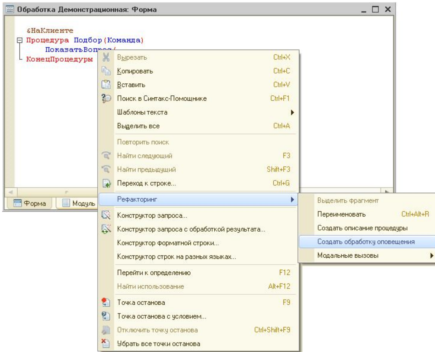
Рис. 175. Создание обработки оповещения с помощью рефакторинга
