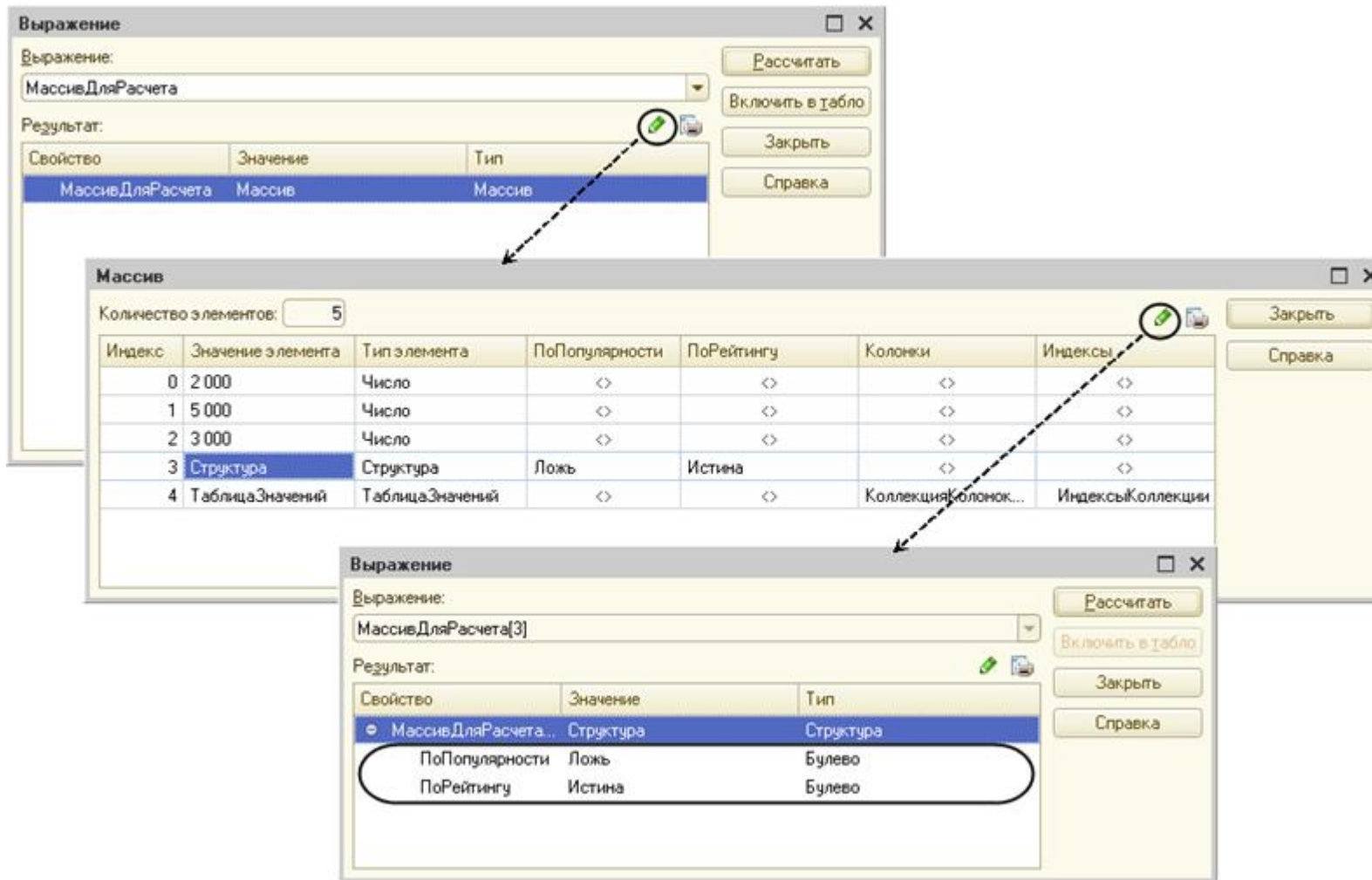
Рис. 155. Просмотр значений коллекции в окне «Выражение»
