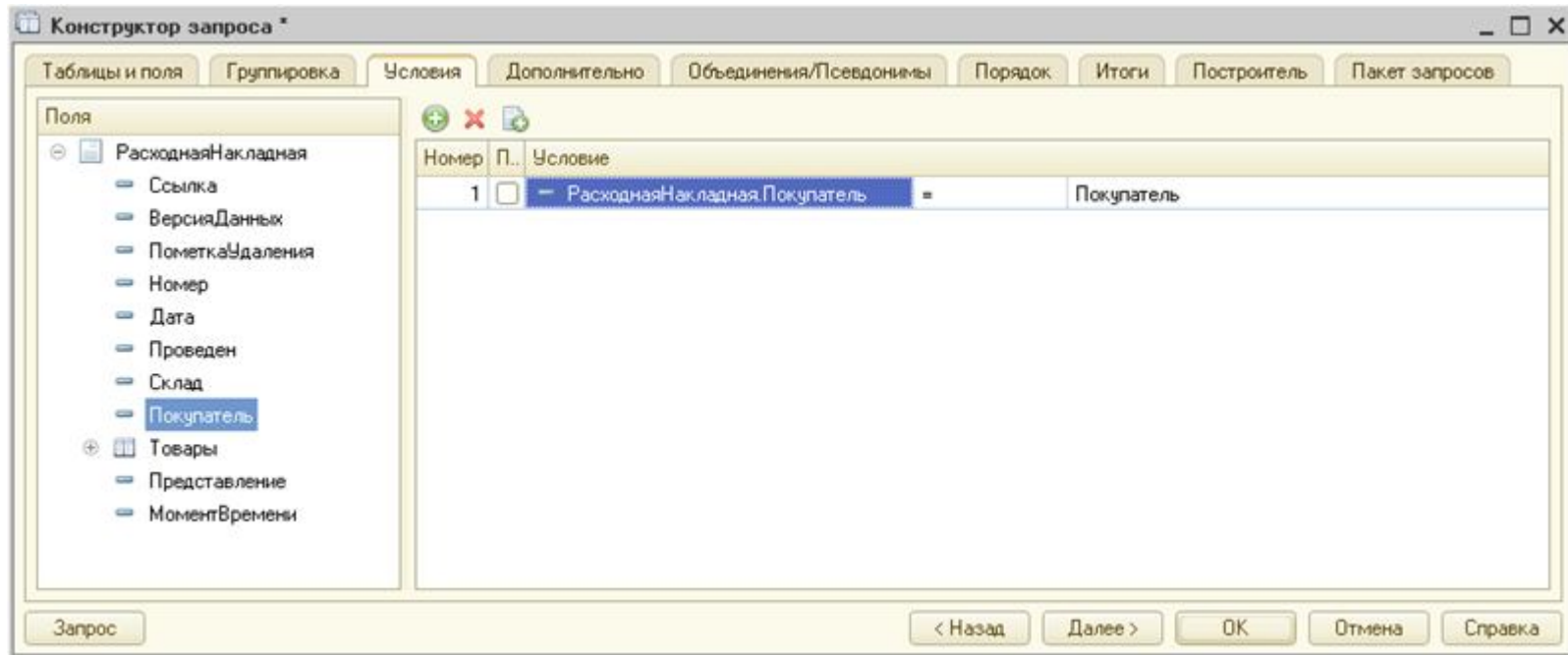
Рис. 141. Условие отбора записей из таблицы
