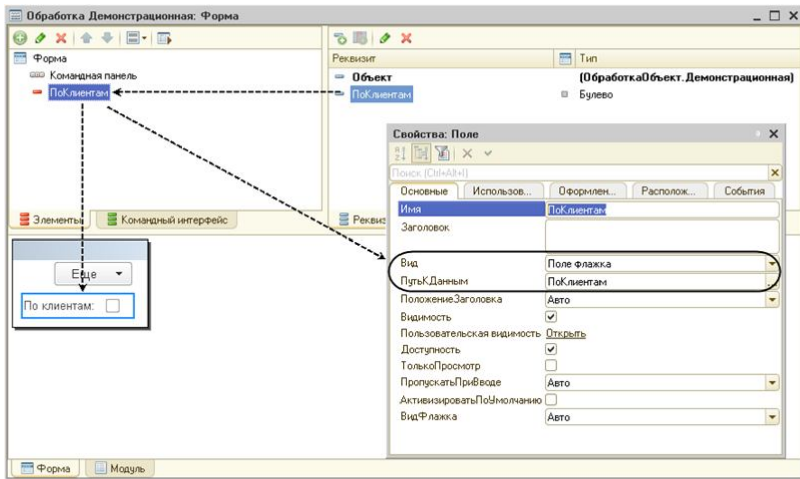
Рис. 90. Создание реквизита формы и связанного с ним поля флажка
