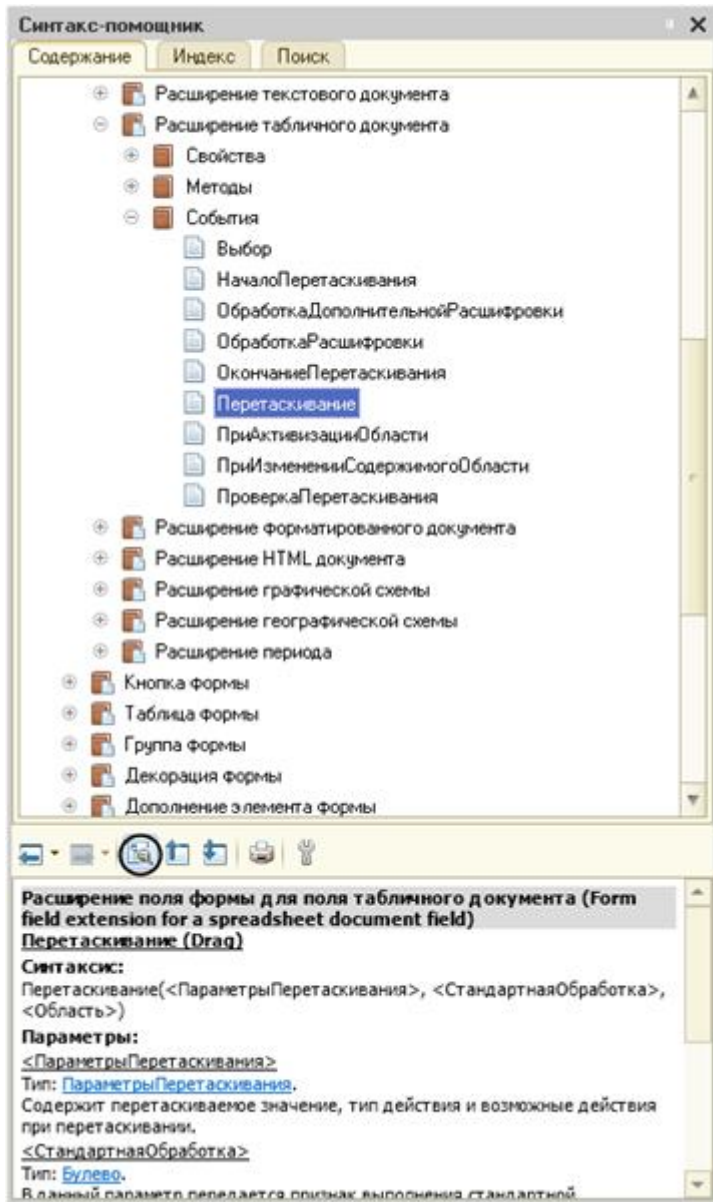
Рис. 29. Переход к текущему описанию в дереве синтаксис-помощника
