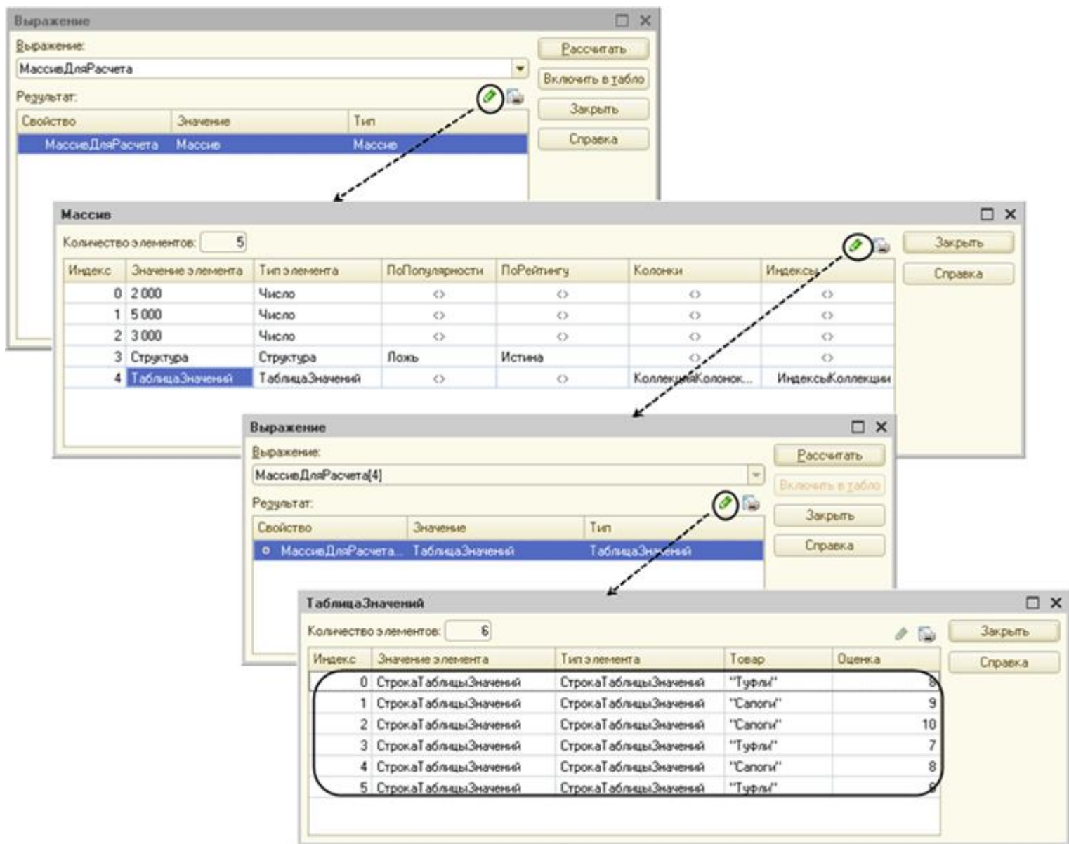
Рис. 156. Просмотр значений коллекции в окне «Выражение»
