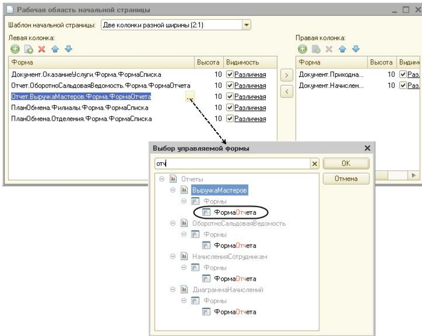
Рис. 60. Поиск форм в окне выбора управляемой формы для заполнения начальной страницы
