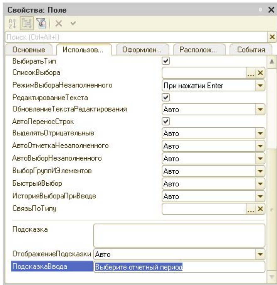
Рис. 105. Установка свойства «ПодсказкаВвода» для поля ввода
