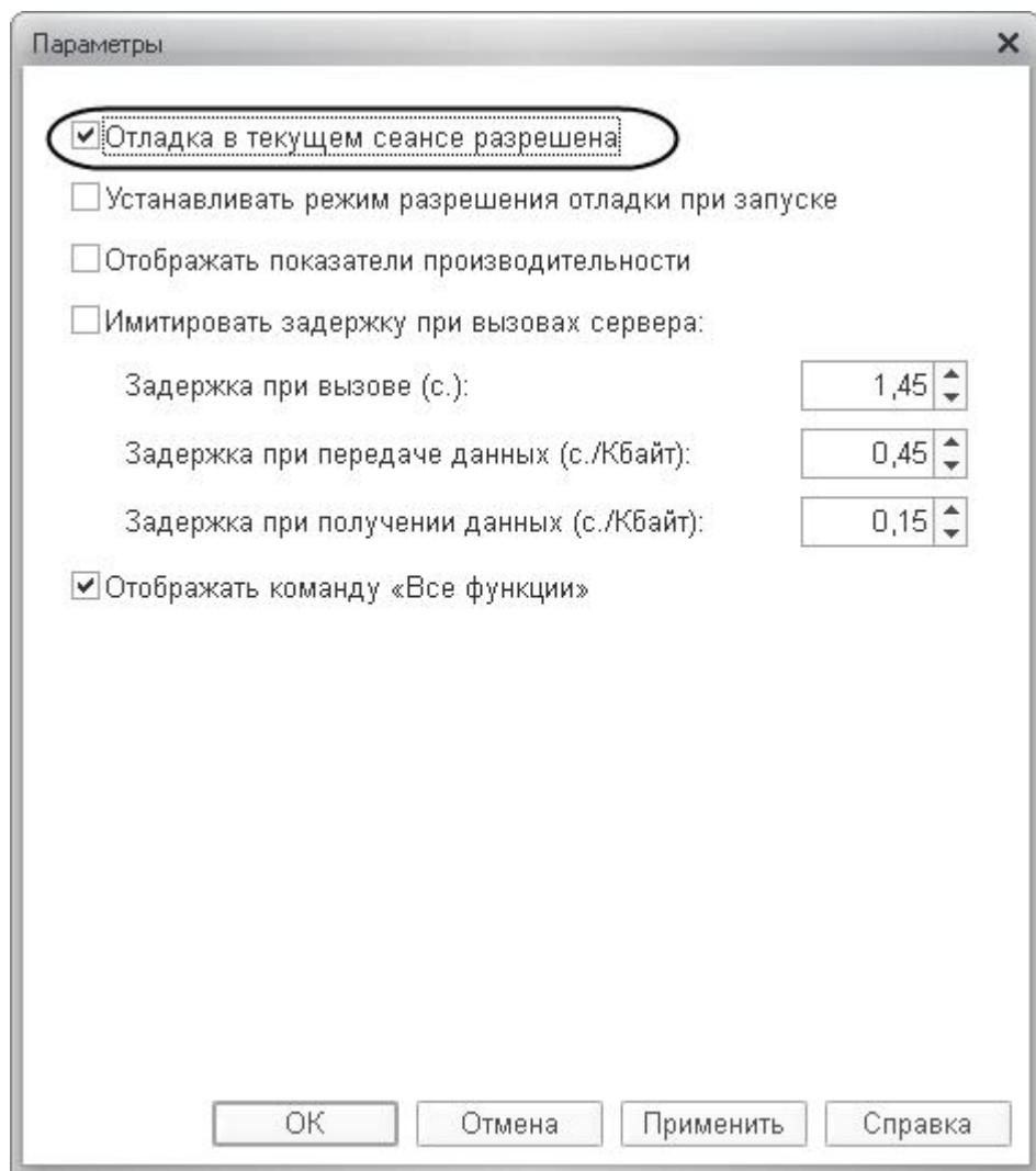
Рис. 151. Установка параметров в режиме «1С:Предприятие»
