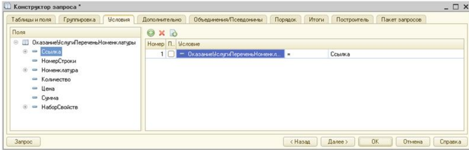
Рис. 136. Условие отбора записей из таблицы
