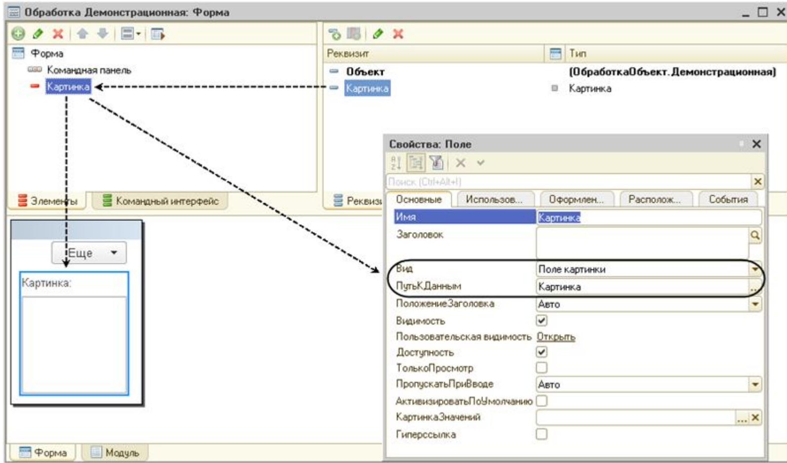
Рис. 91. Создание реквизита формы и связанного с ним поля картинки
