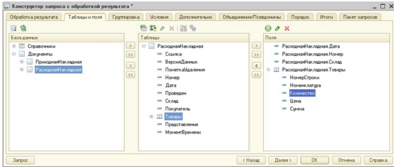
Рис. 140. Исходные данные для запроса
