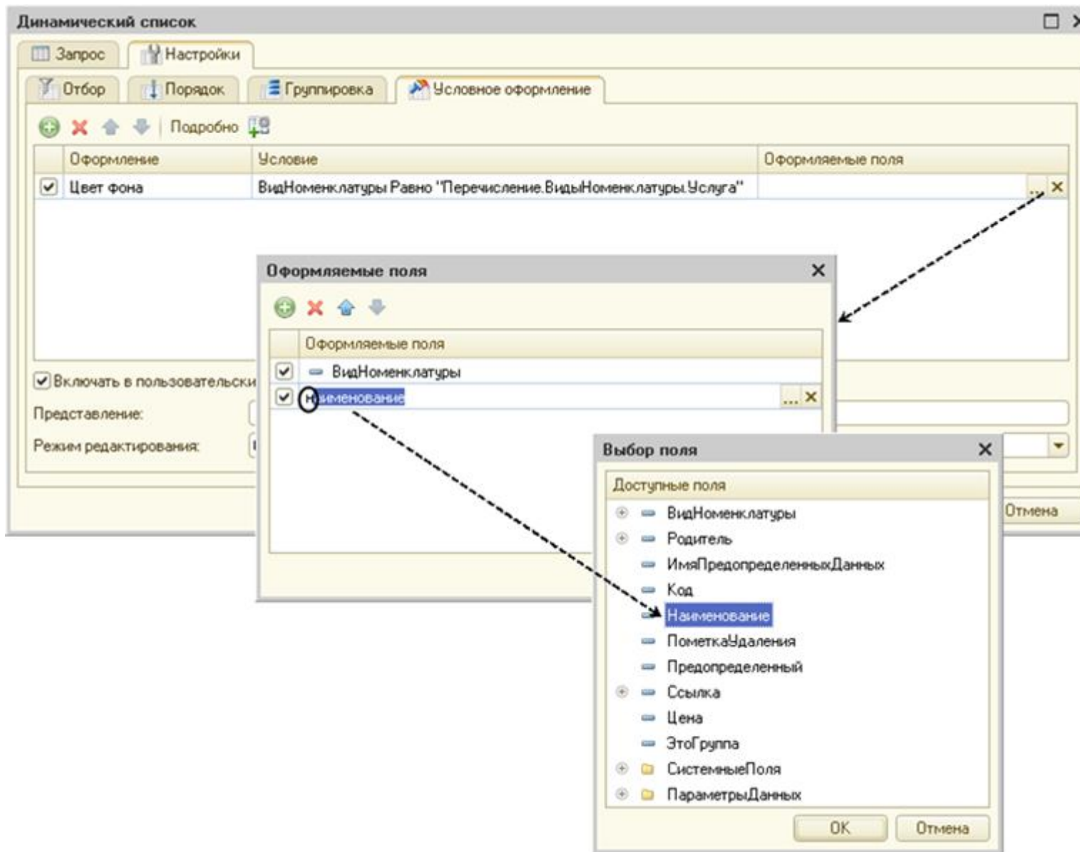
Рис. 184. Выбор полей в настройках динамического списка
