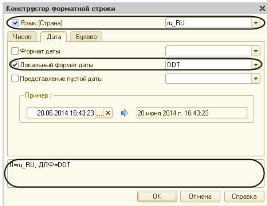
Рис. 129. Конструктор форматной строки
