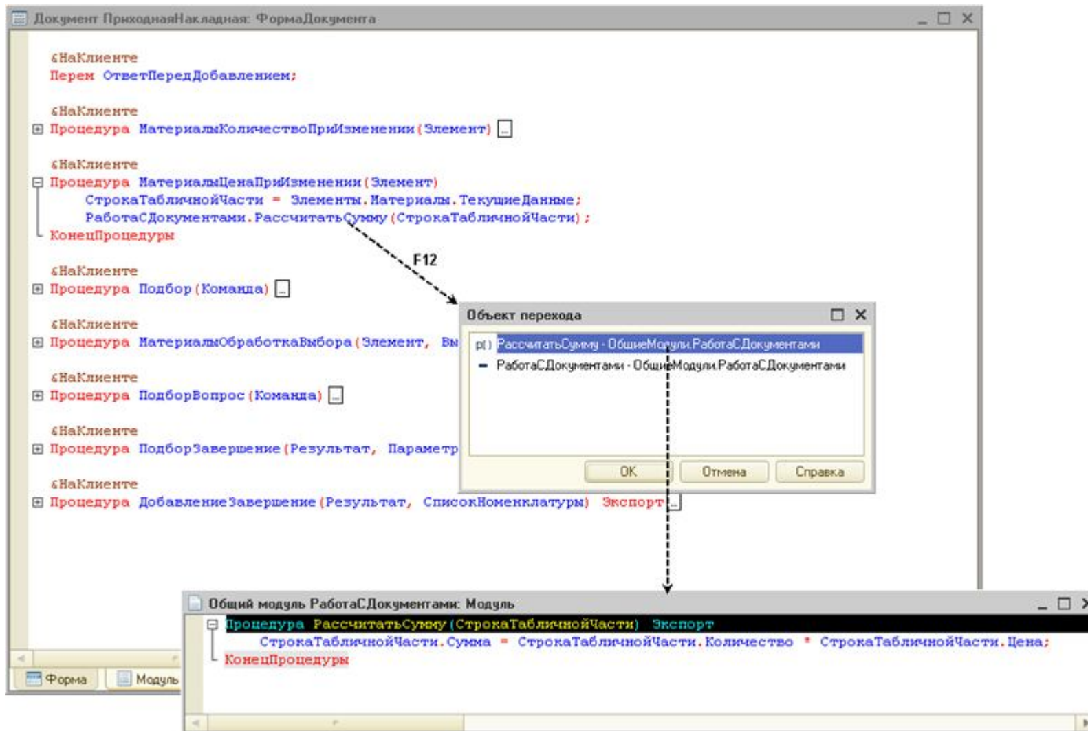
Рис. 69. Переход к определению процедуры или функции
