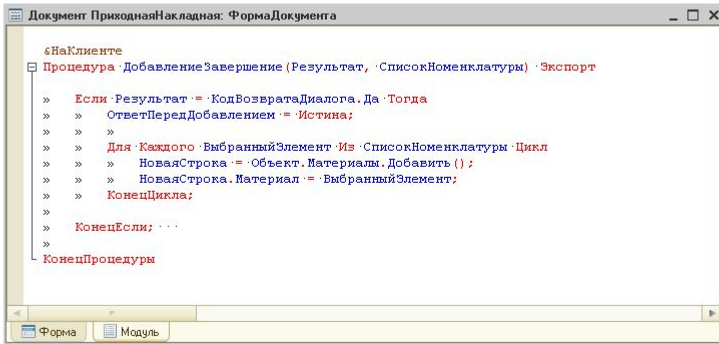
Рис. 12. Отображение непечатаемых символов в тексте модуля
