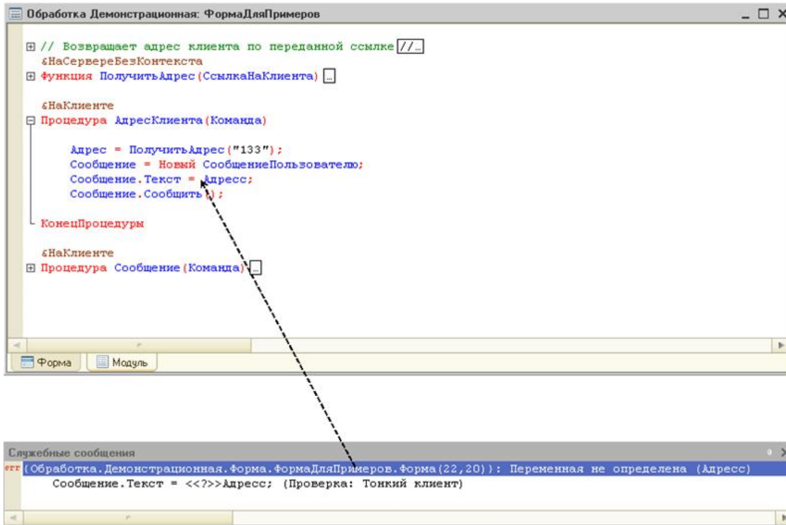
Рис. 52. Переход к строке с ошибкой из окна сообщения об ошибках
