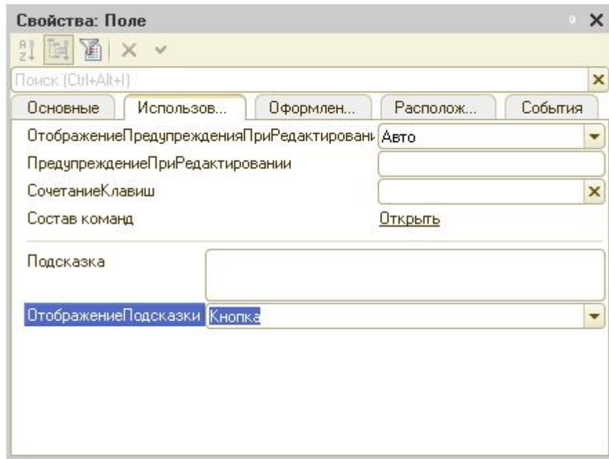
Рис. 107. Установка свойства «ОтображениеПодсказки» для поля флажка
