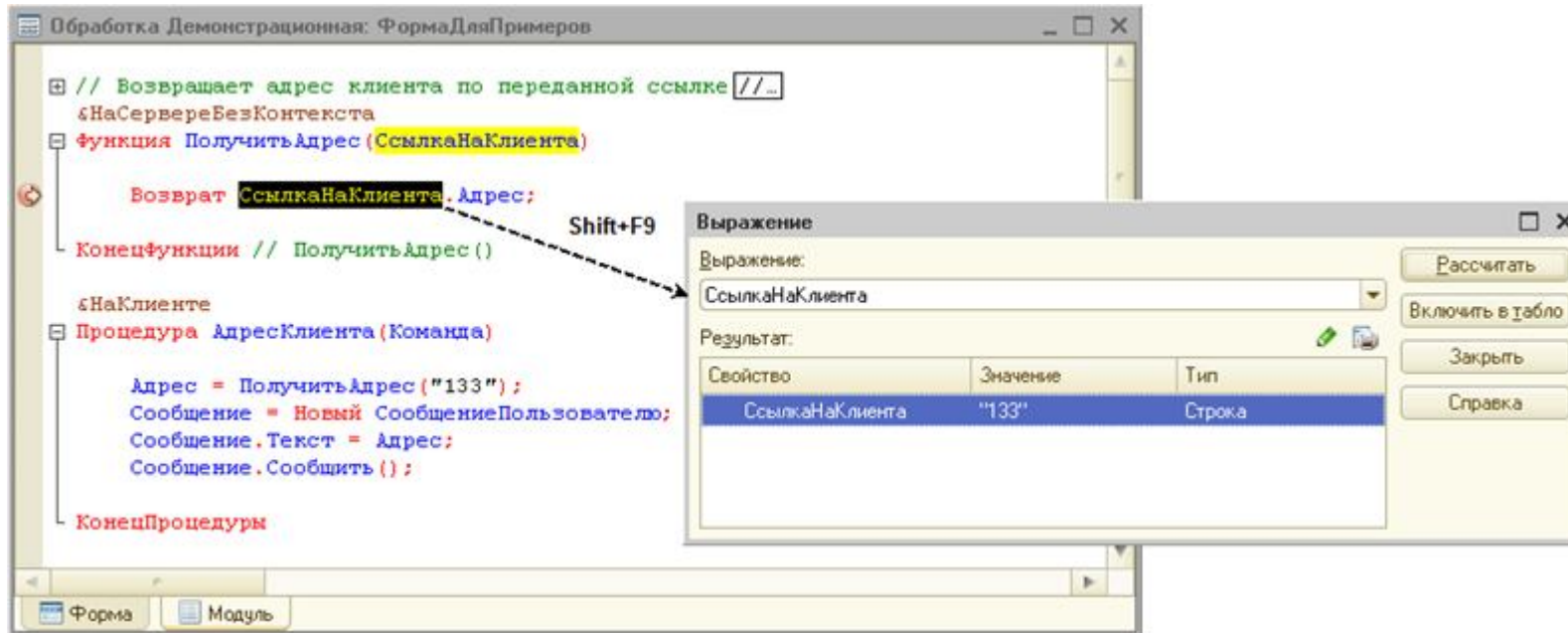
Рис. 165. Просмотр значения параметра при передаче в функцию
