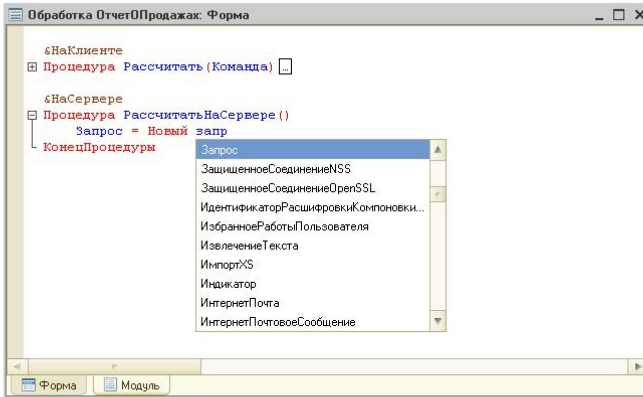
Рис. 120. Создание объекта «Запрос»
