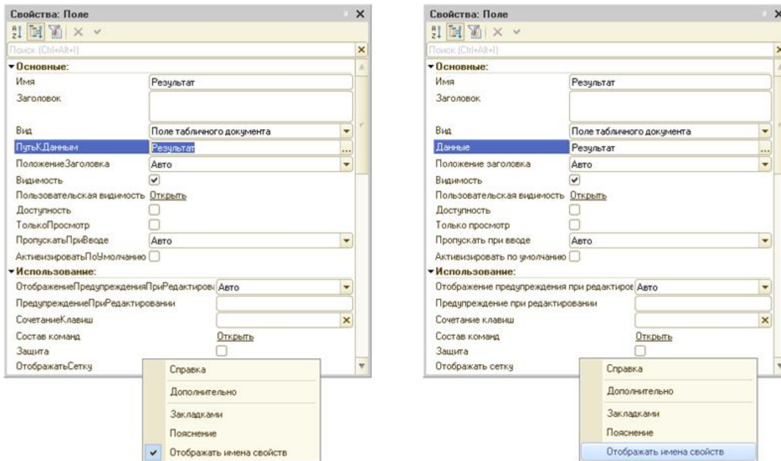
Рис. 43. Режим отображения имен/представлений свойств
