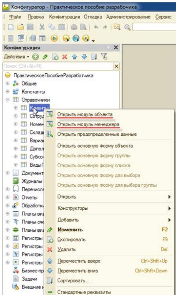
Рис. 56. Модули объектов
