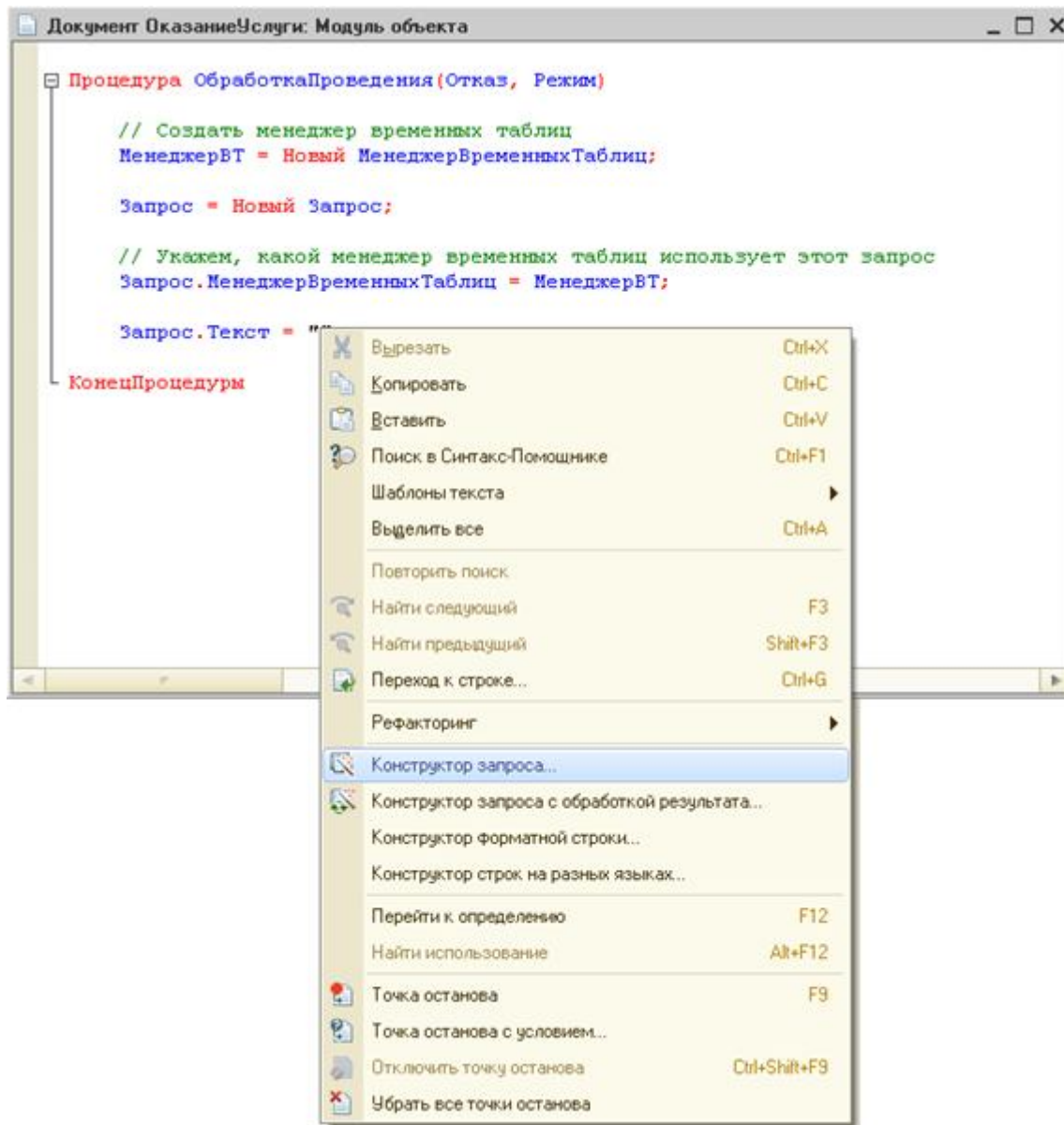
Рис. 134. Вызов конструктора запроса
