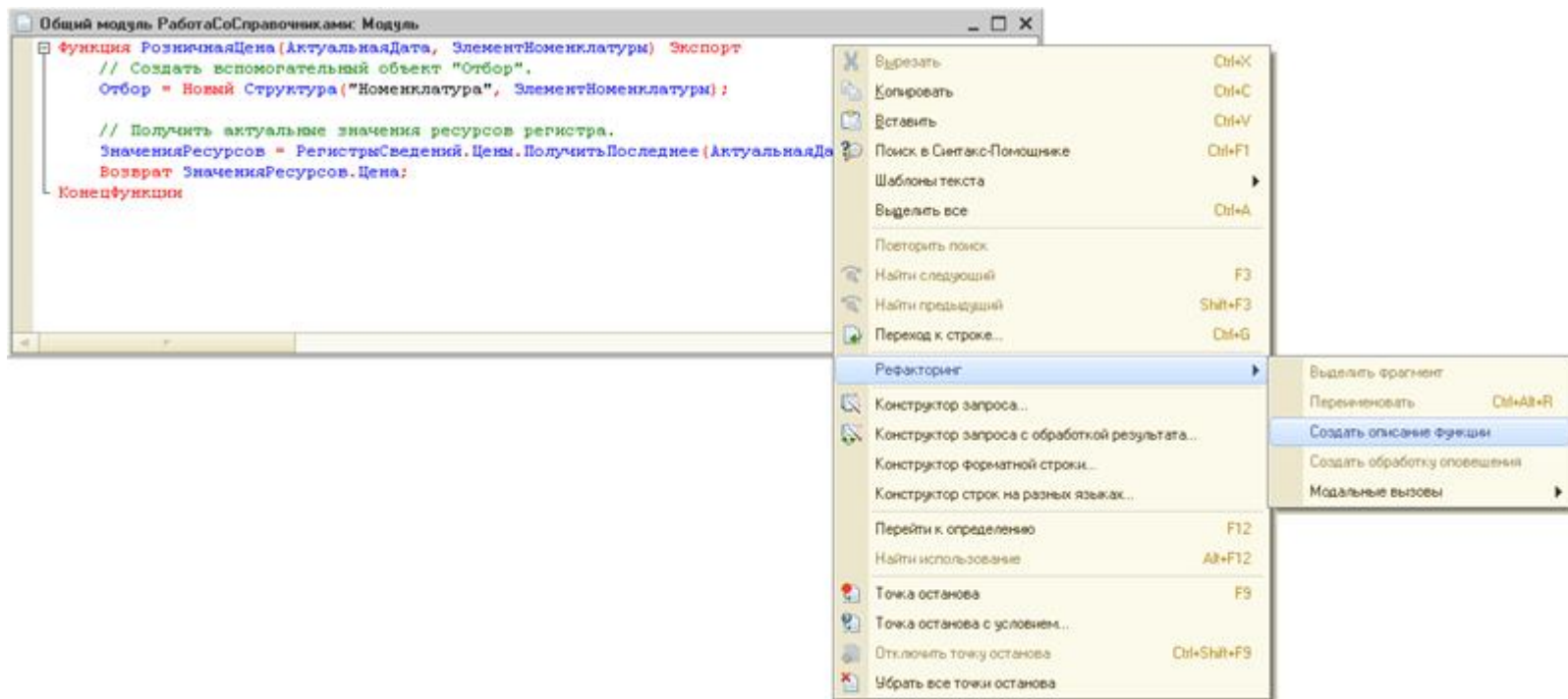
Рис. 174. Создание описания функции с помощью рефакторинга
