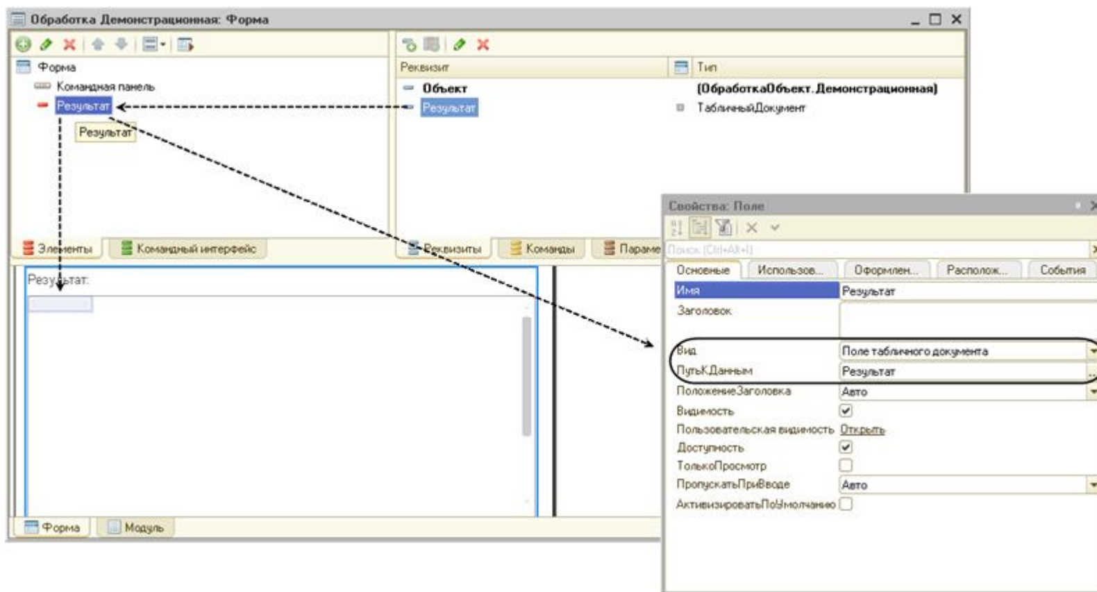
Рис. 88. Создание реквизита формы и связанного с ним поля табличного документа
