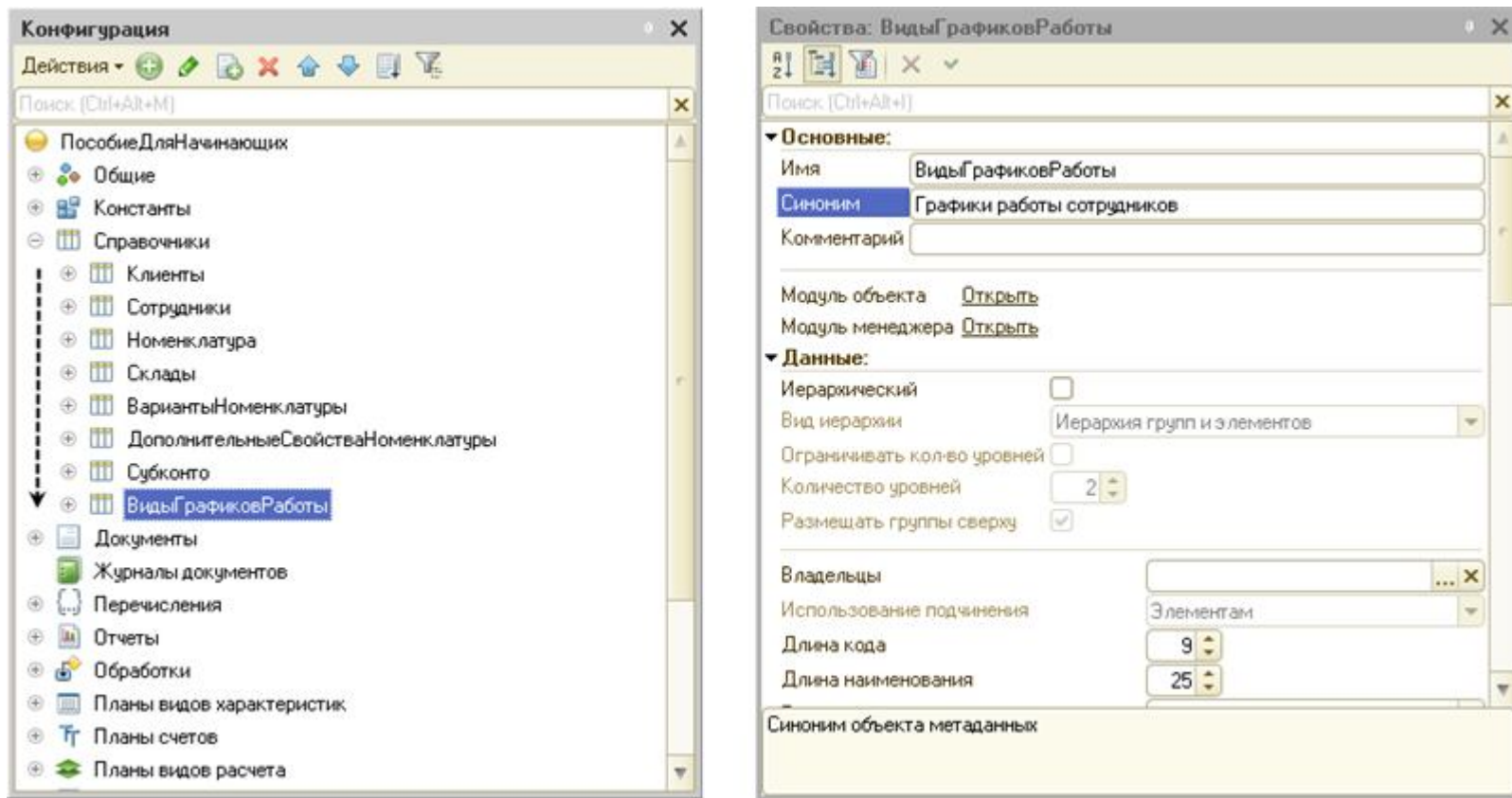
Рис. 39. Палитра свойств текущего объекта конфигурации
