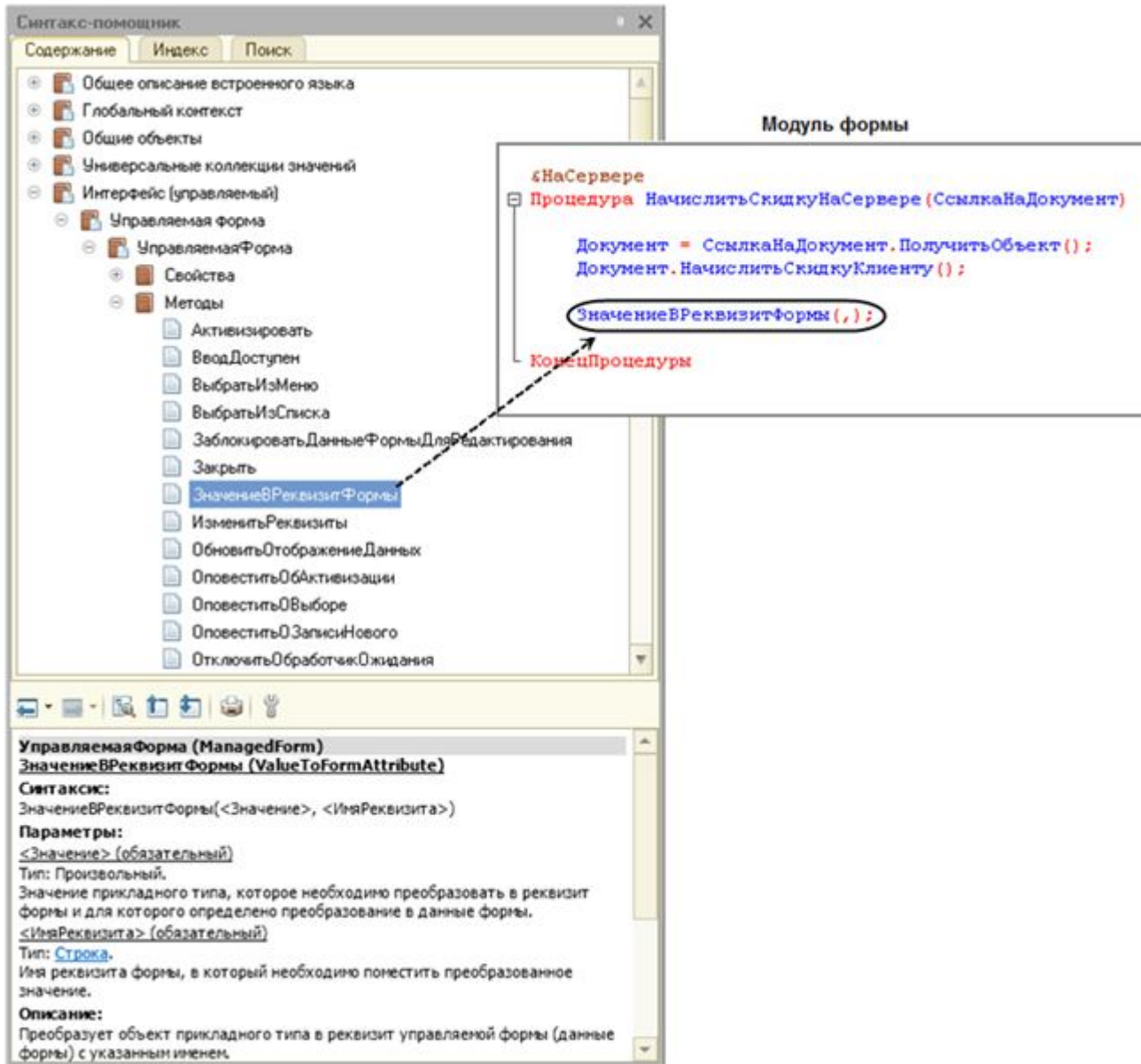
Рис. 81. Перетаскивание свойств, методов из синтаксис-помощника
