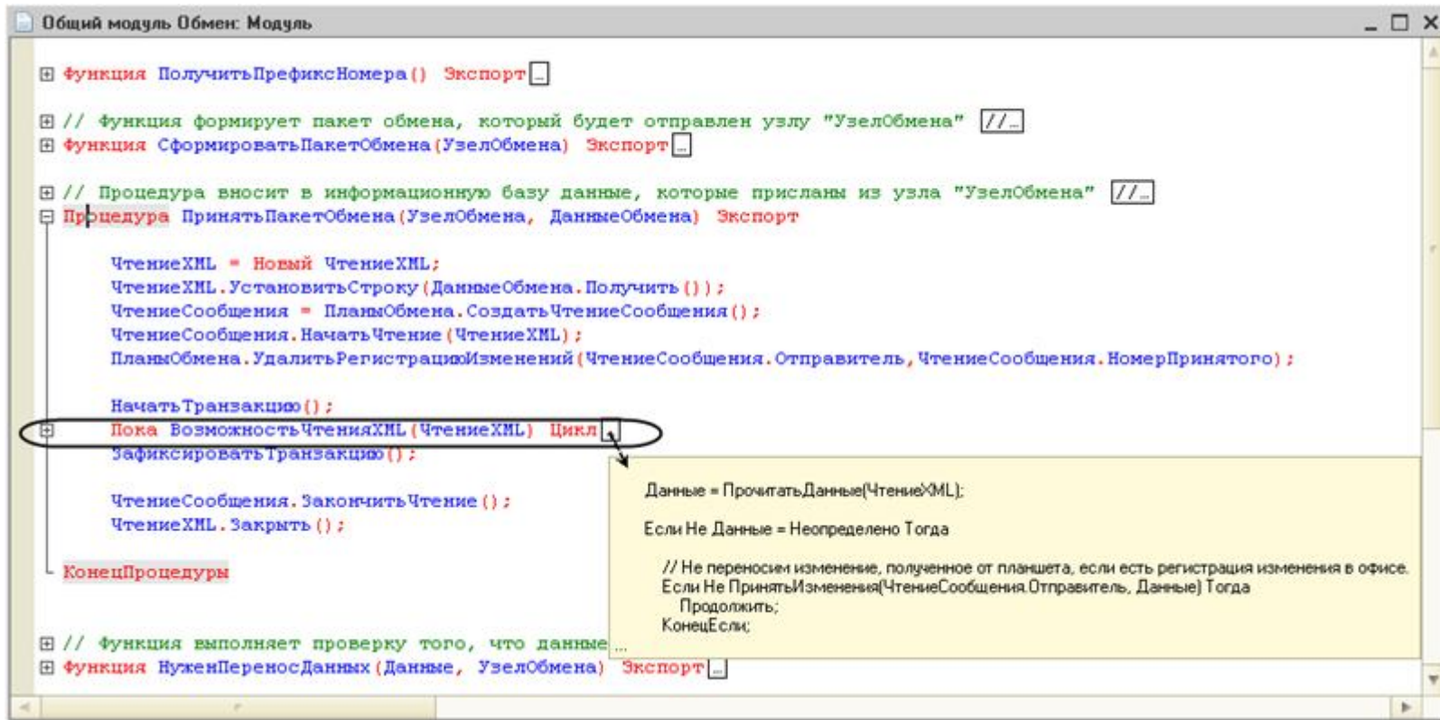
Рис. 22. Вид свернутых и развернутых групп в тексте модуля
