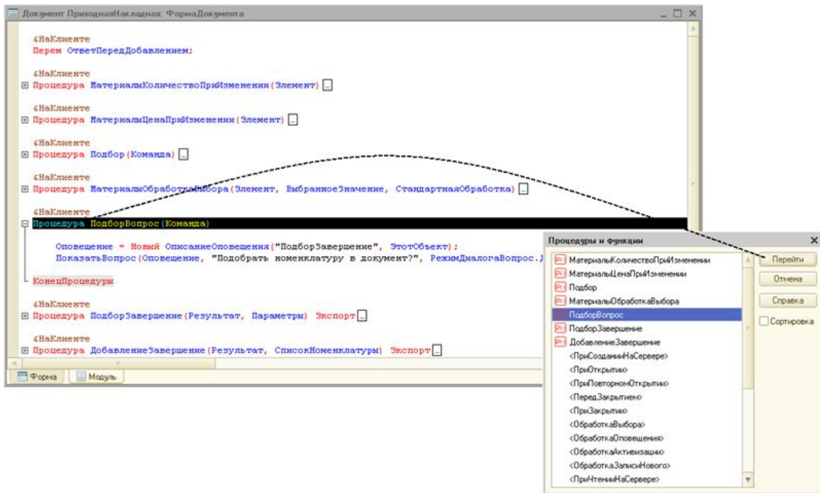
Рис. 67. Окно «Процедуры и функции»
