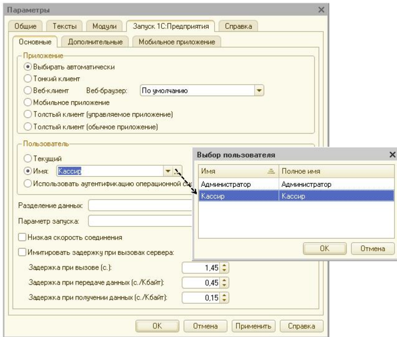
Рис. 149. Выбор пользователя, от имени которого будет запускаться «1С:Предприятие»
