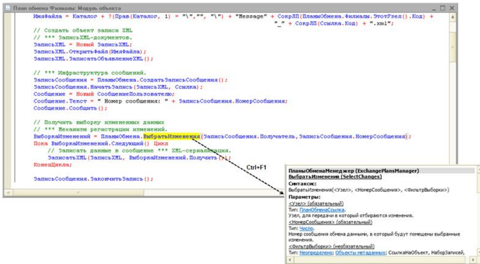
Рис. 28. Использование контекстной помощи синтакс-помощника
