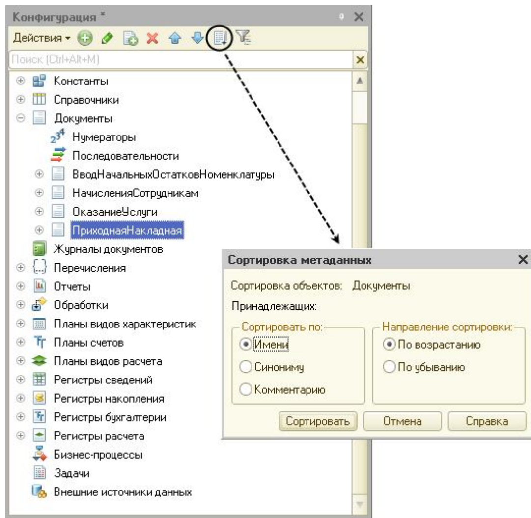
Рис. 37. Сортировка объектов в дереве объектов конфигурации
