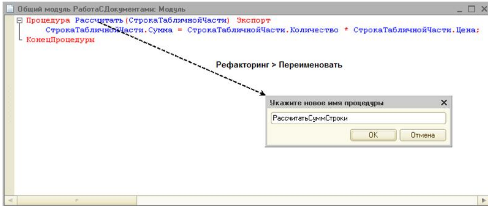
Рис. 171. Переименование экспортируемой процедуры общего модуля
