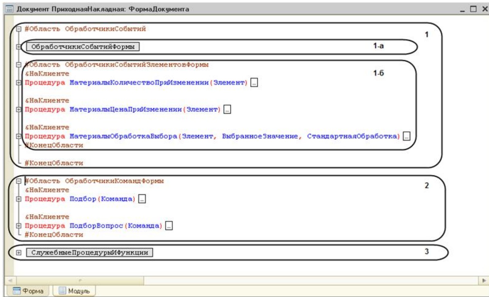
Рис. 23. Модуль формы с выделенными разделами в виде областей
