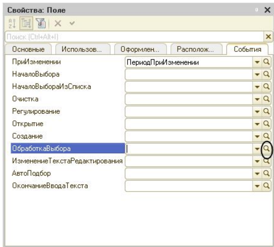
Рис. 103. Создание обработчика события из палитры свойств элемента формы
