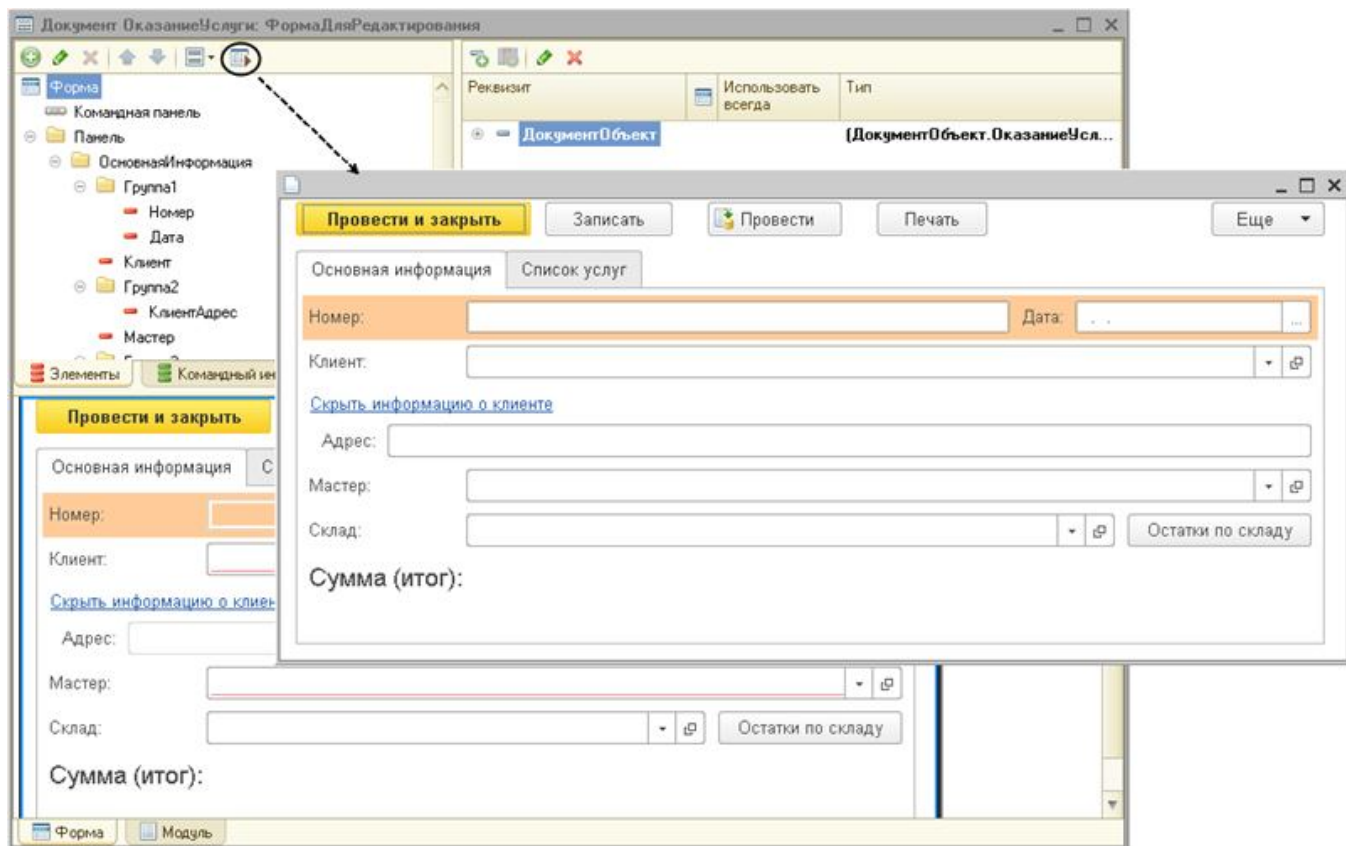
Рис. 62. Вид формы в интерфейсе приложения
