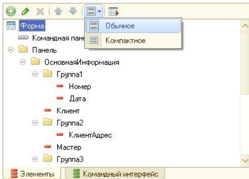
Рис. 63. Переключение режимов отображения в редакторе формы
