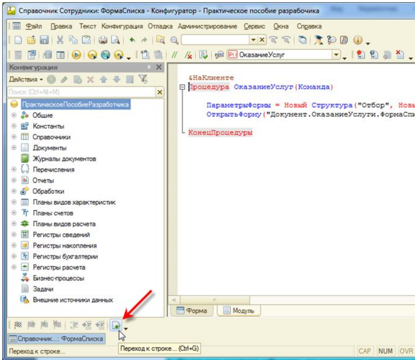
Рис. 58. Переход к строке
