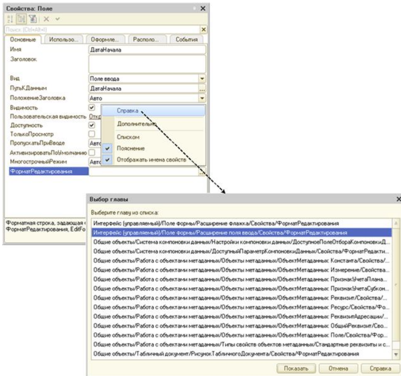
Рис. 30. Вызов синтакс-помощника из палитры свойств
