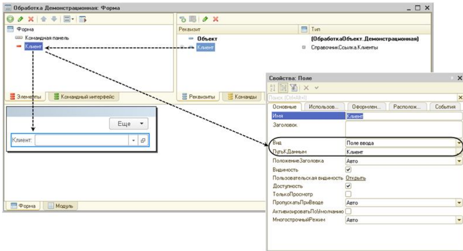
Рис. 87. Создание реквизита формы и связанного с ним поля ввода
