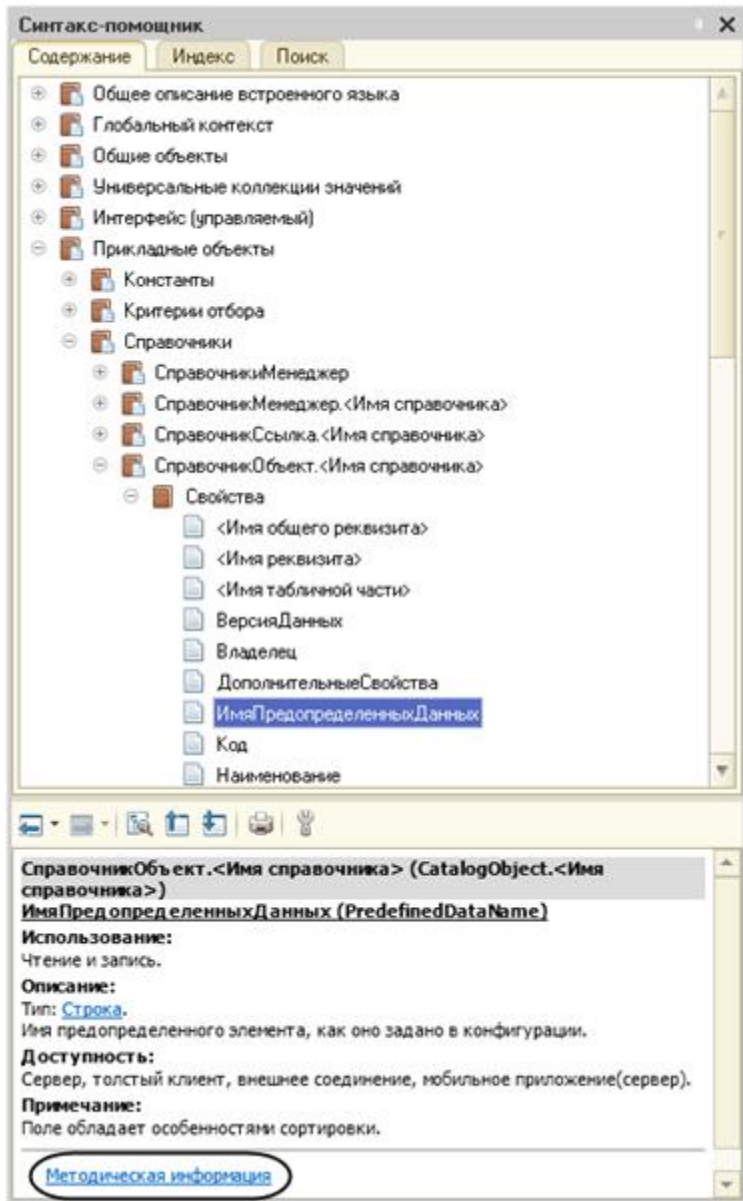
Рис. 31. Переход к методической информации из синтаксис-помощника
