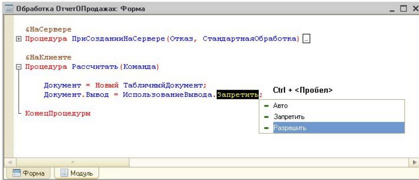
Рис. 117. Изменение значений перечисления с помощью контекстной подсказки
