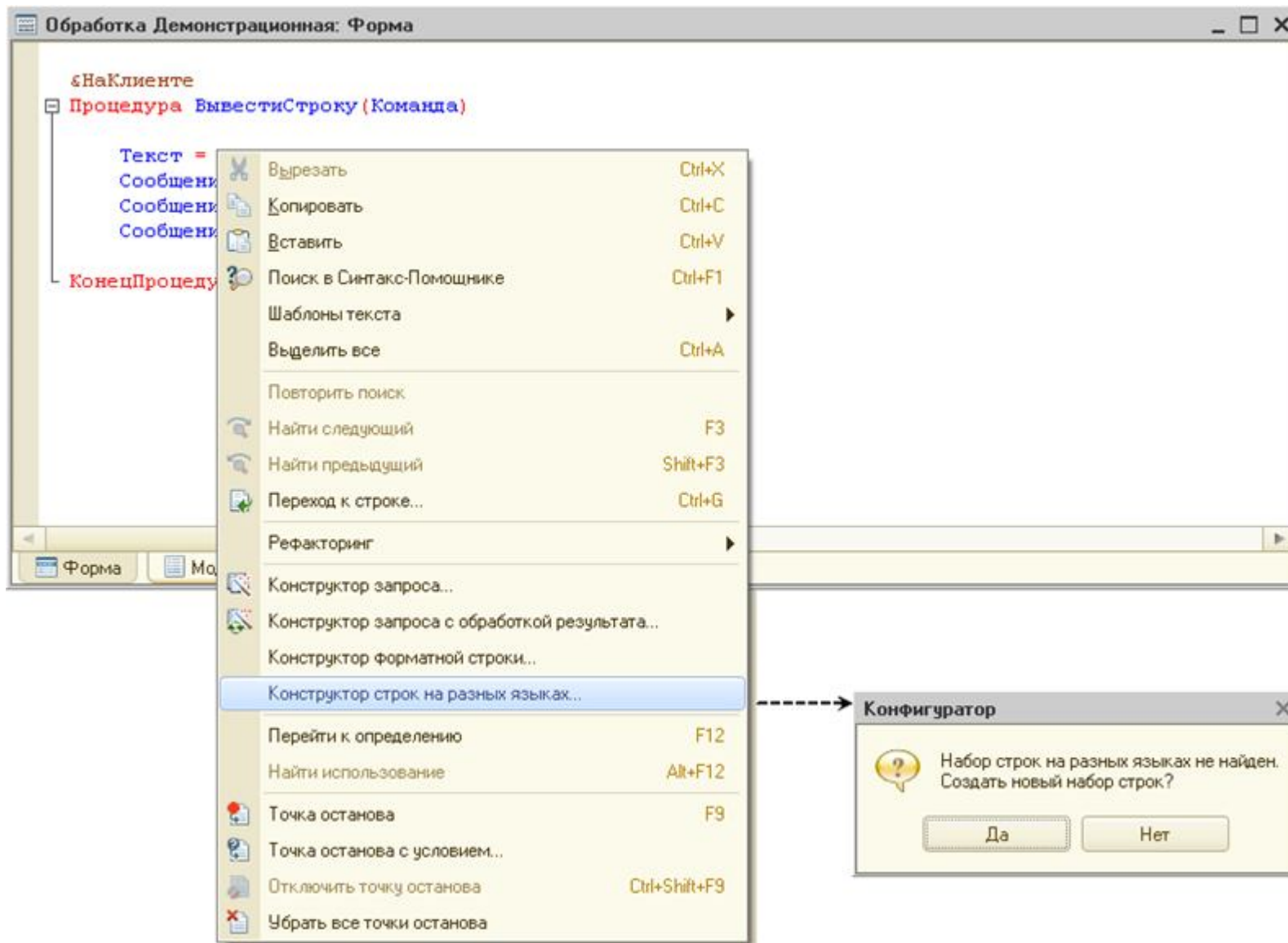
Рис. 177. Вызов конструктора строк на разных языках
