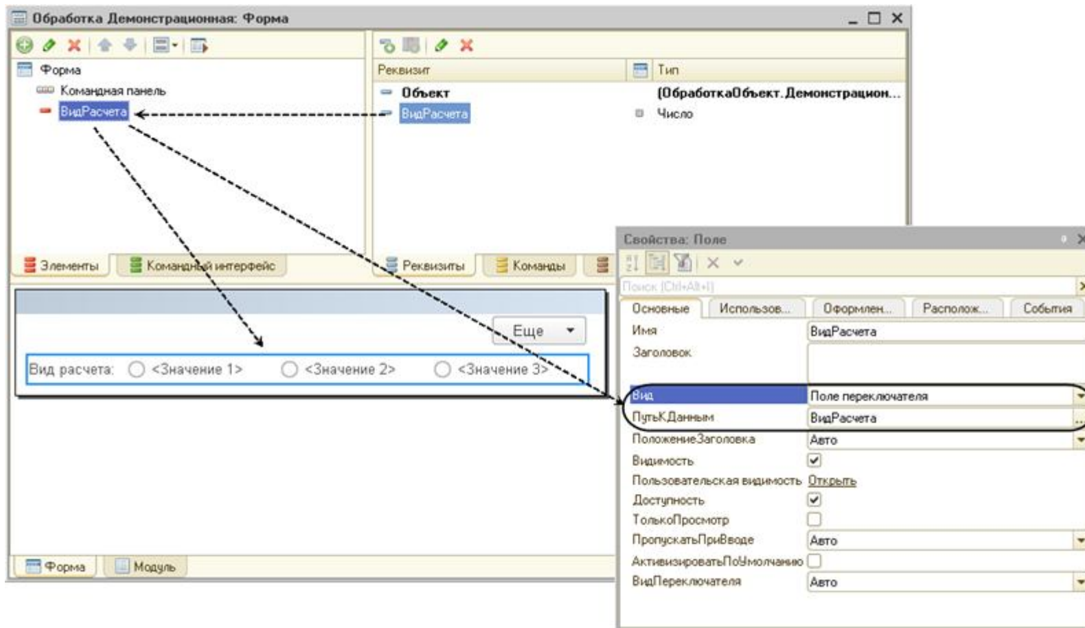
Рис. 92. Создание реквизита формы и связанного с ним поля переключателя
