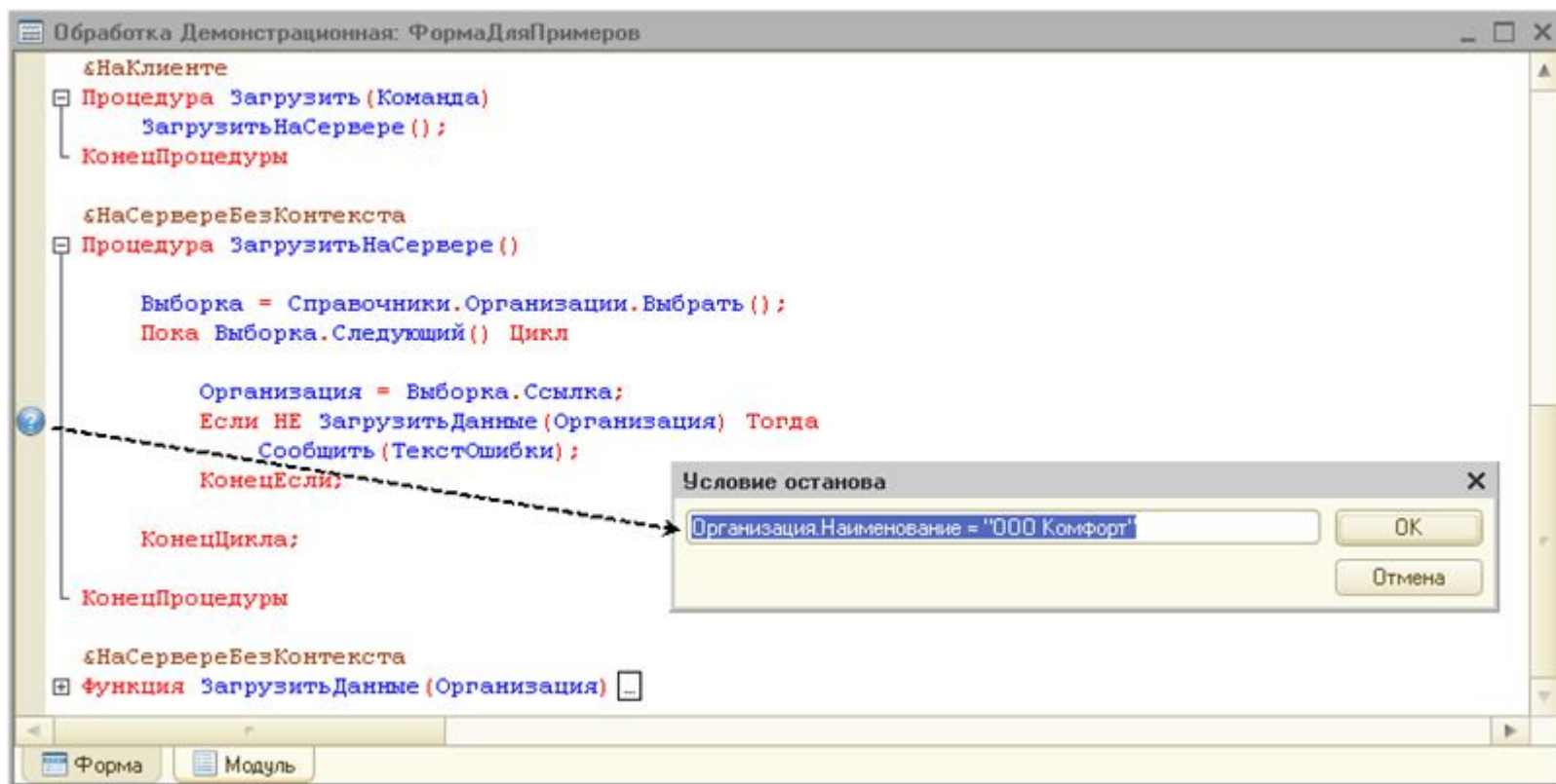
Рис. 161. Установка условия останова
