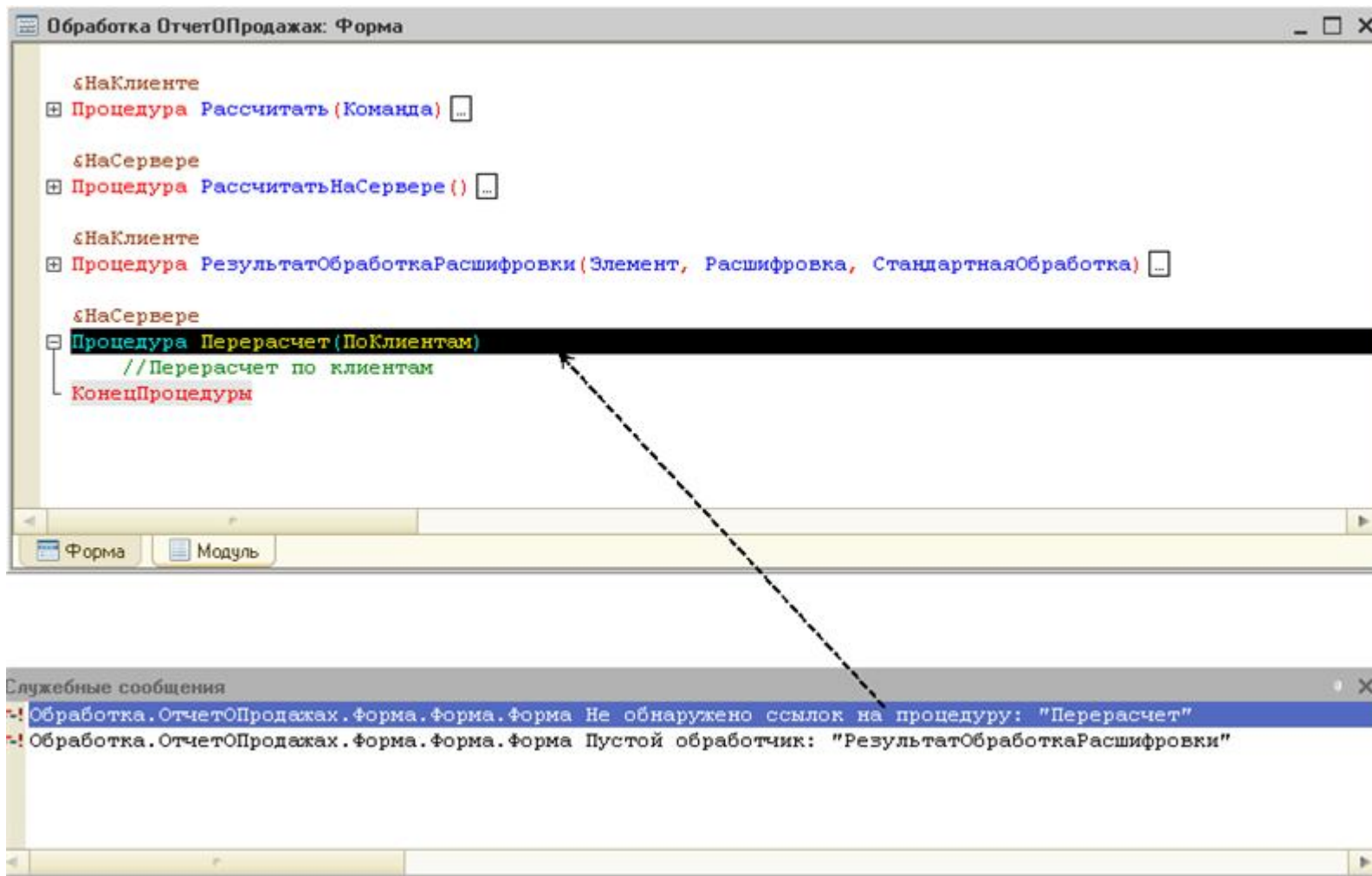
Рис. 189. Переход к ошибке, найденной при проверке конфигурации
