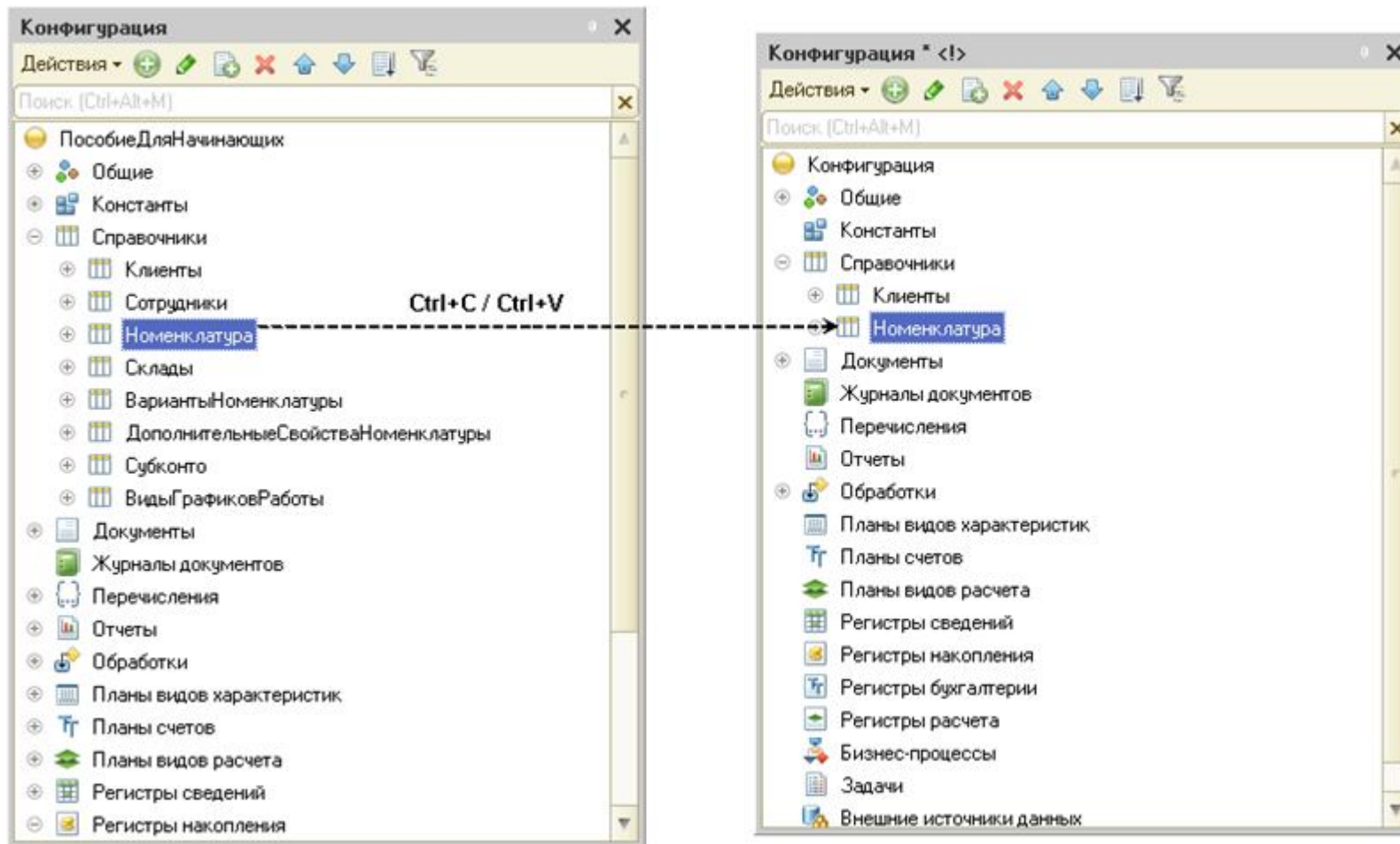
Рис. 74. Копирование объектов между разными конфигурациями
