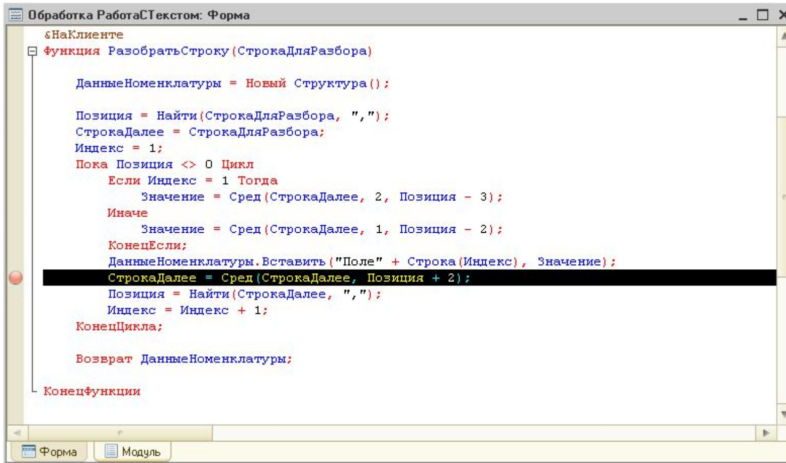
Рис. 162. Установка точки останова в цикле разбора строки
