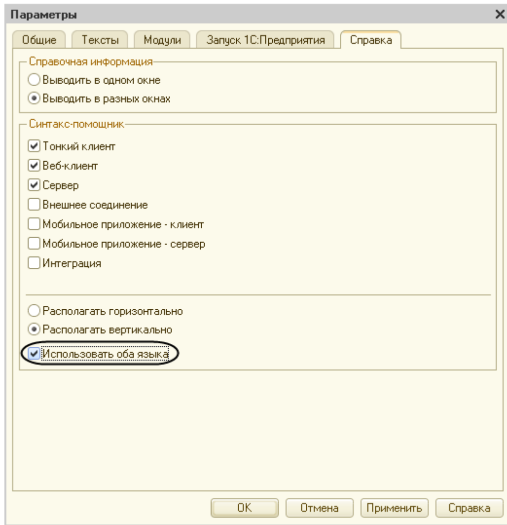
Рис. 18. Настройка параметров синтакс-помощника
