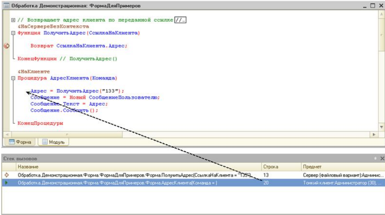
Рис. 166. Переход из окна стека вызовов к нужной процедуре
