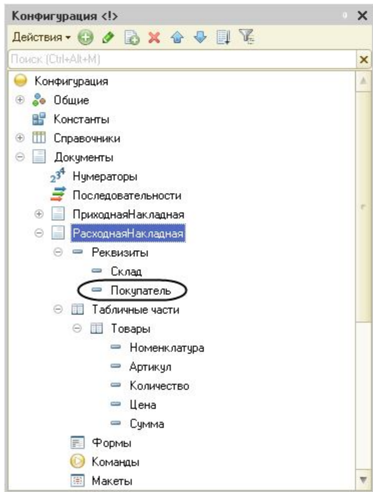
Рис. 72. Копирование объекта в дереве объектов конфигурации
