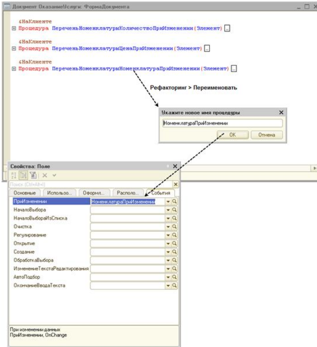
Рис. 172. Переименование процедуры – обработчика события в модуле формы и в палитре свойств
