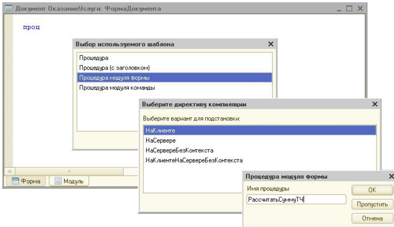
Рис. 122. Создание шаблона процедуры в модуле формы с помощью автозамены
