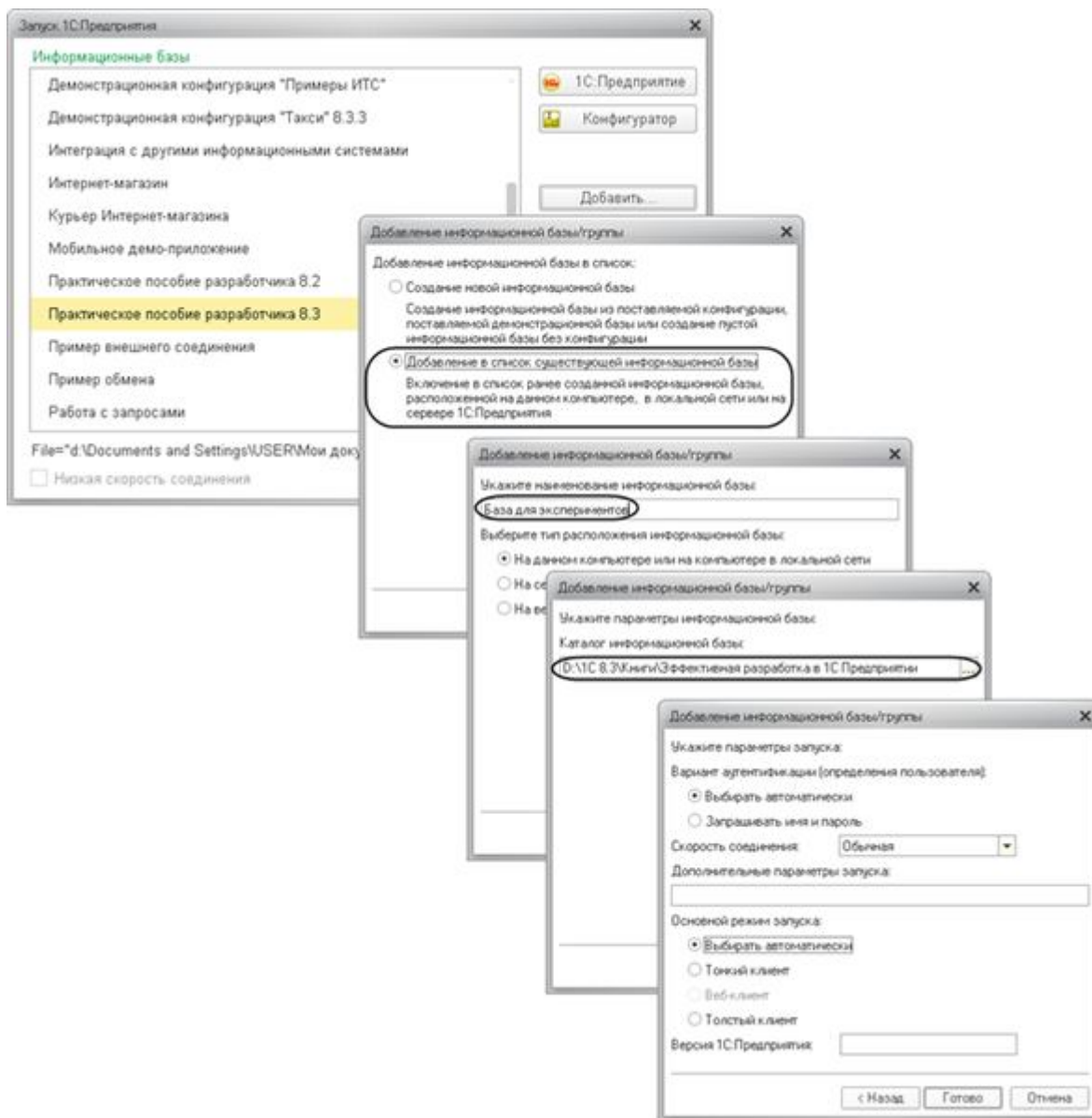
Рис. 85. Добавление в список информационных баз «1С:Предприятия» существующей информационной базы
