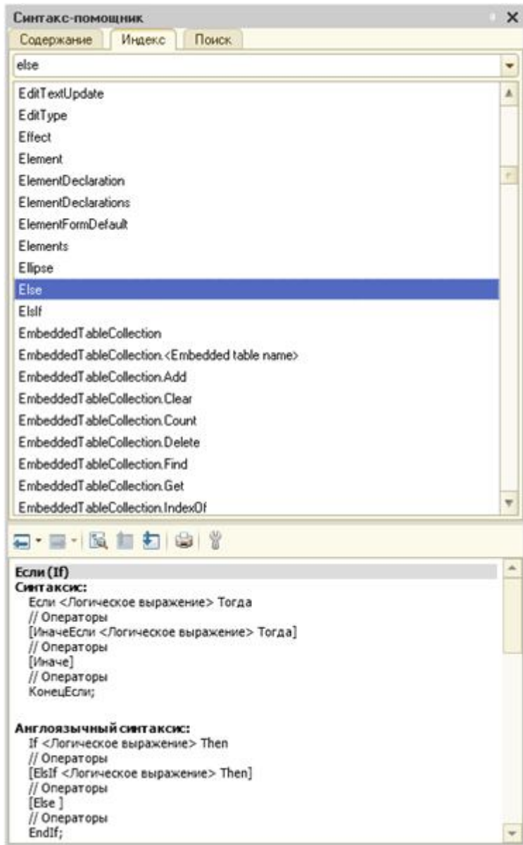
Рис. 19. Окно синтаксис-помощника
