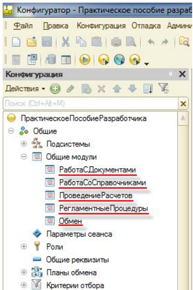
Рис. 55. Общие модули
