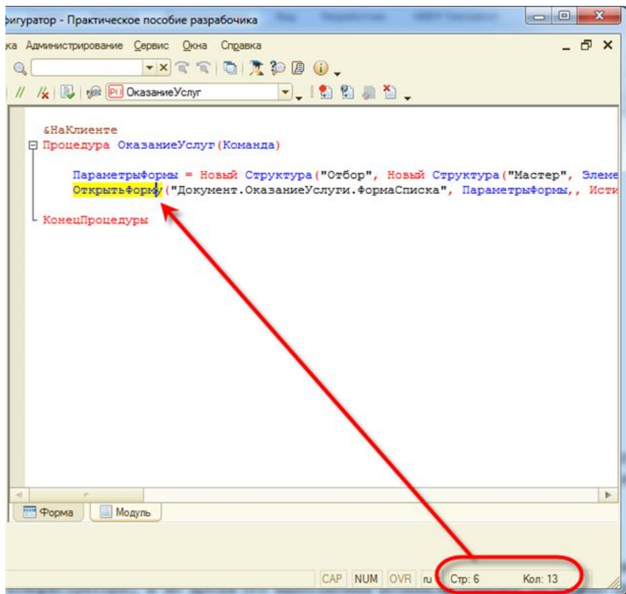
Рис. 59. Позиция курсора
