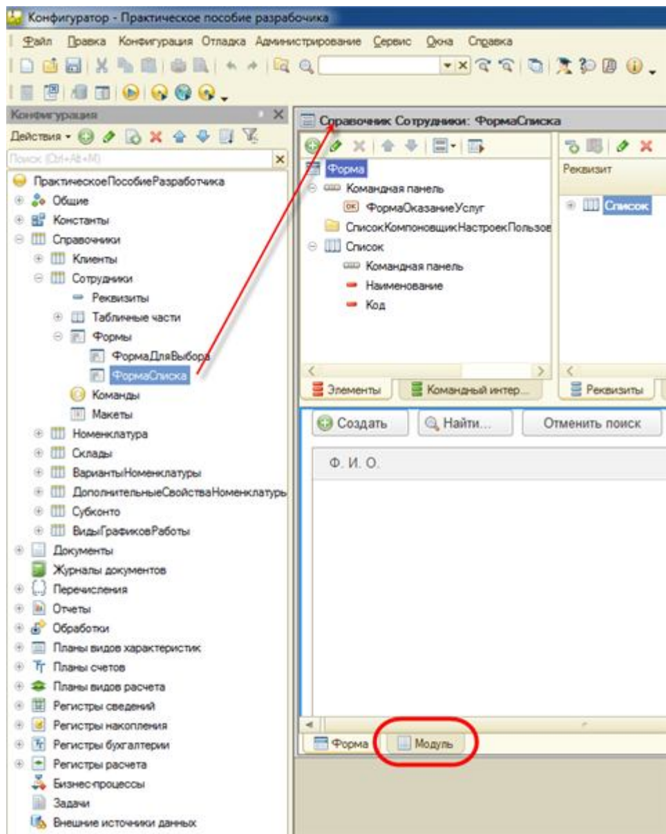
Рис. 57. Модуль формы
