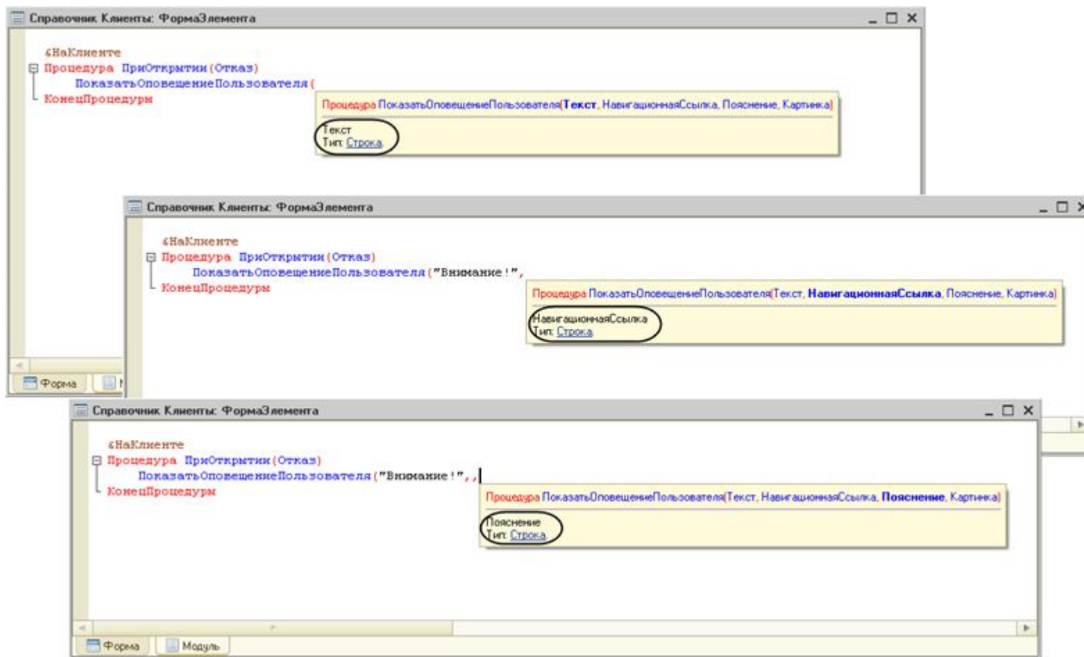
Рис. 118. Использование контекстной подсказки при написании параметров процедуры
