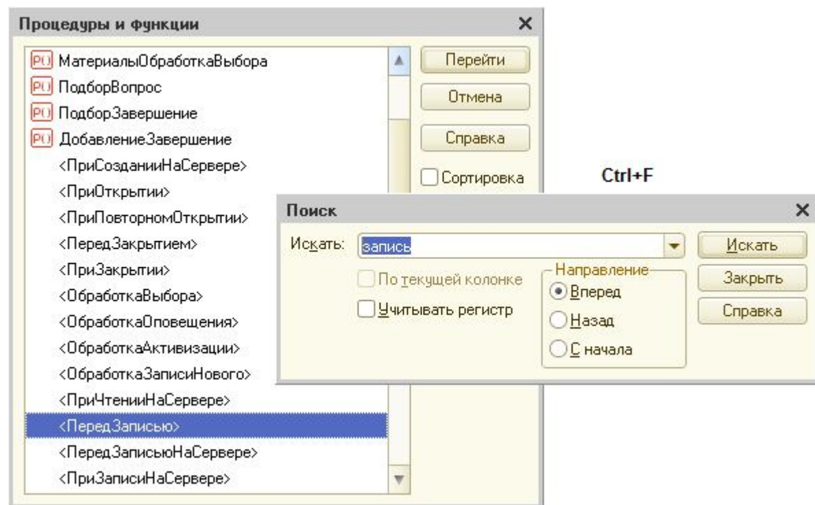
Рис. 68. Выпадающий список процедур и функций модуля
