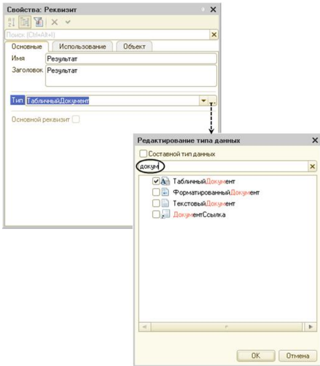
Рис. 89. Поиск типов объектов в строке поиска при выборе типа
