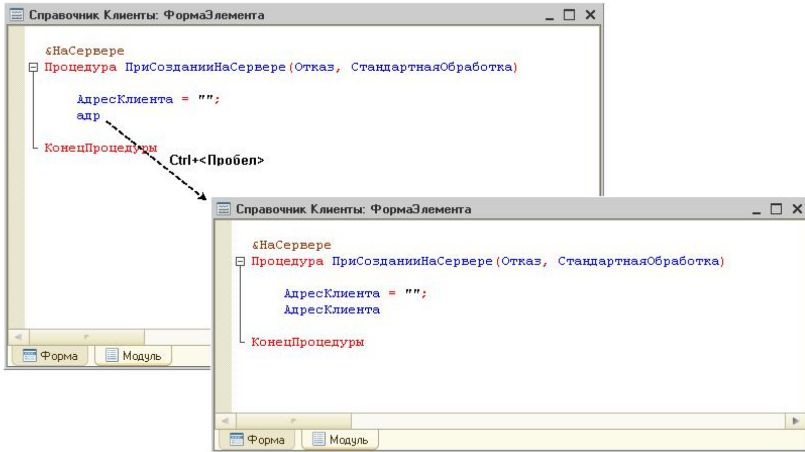
Рис. 111. Использование контекстной подсказки при написании имени переменной
