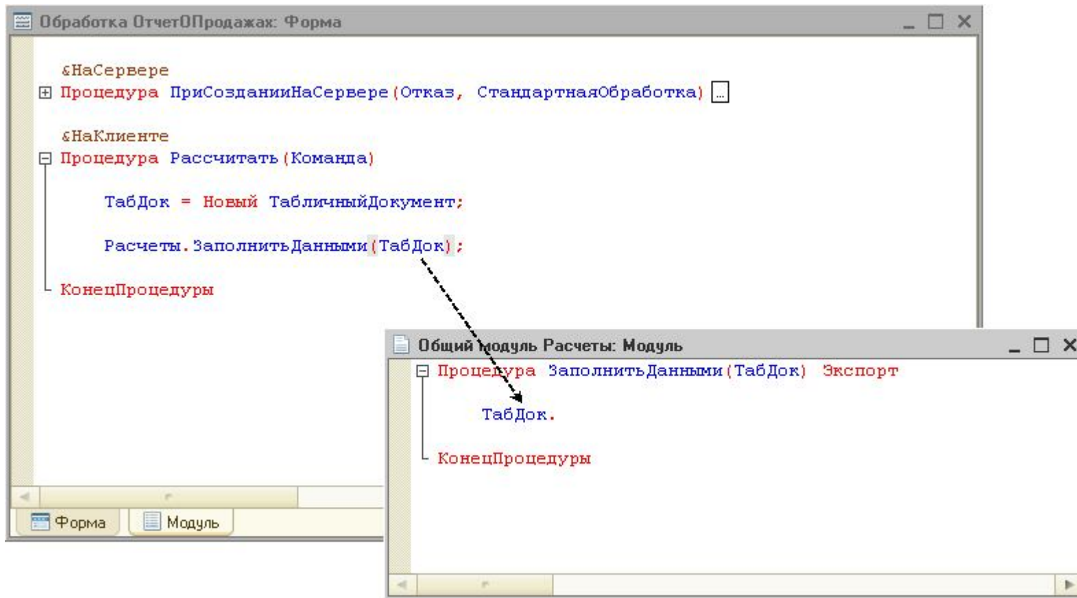
Рис. 27. Отсутствие контекстной подсказки для табличного документа, переданного в процедуру общего модуля в качестве параметра
