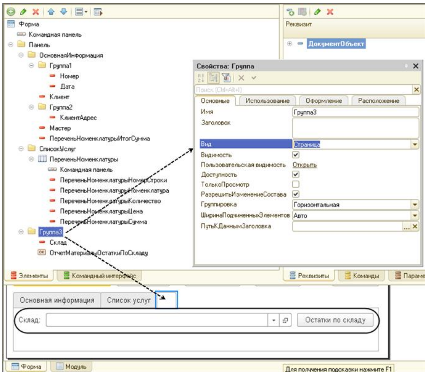
Рис. 79. Перетаскивание элементов формы
