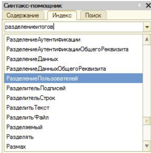
Рис. 33. Попытка поиска по индексу в синтакс-помощнике
