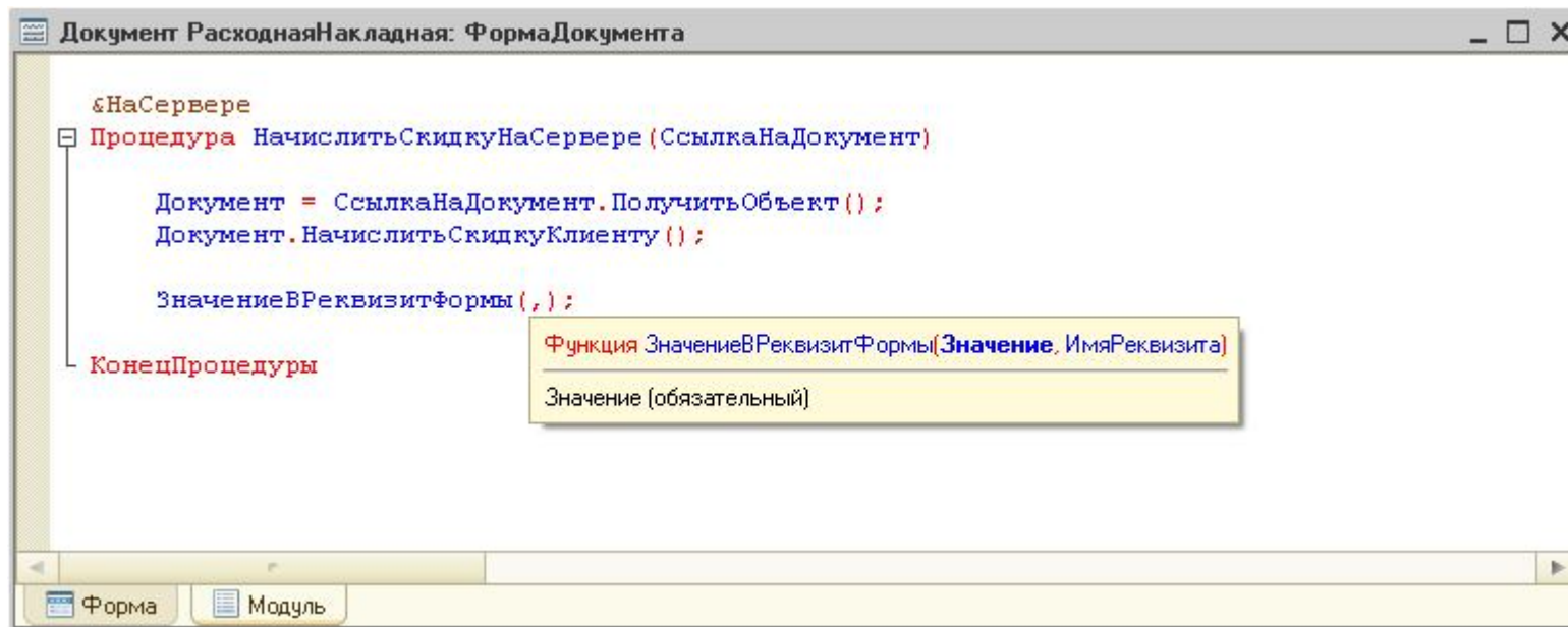
Рис. 82. Вызов контекстной подсказки параметров
