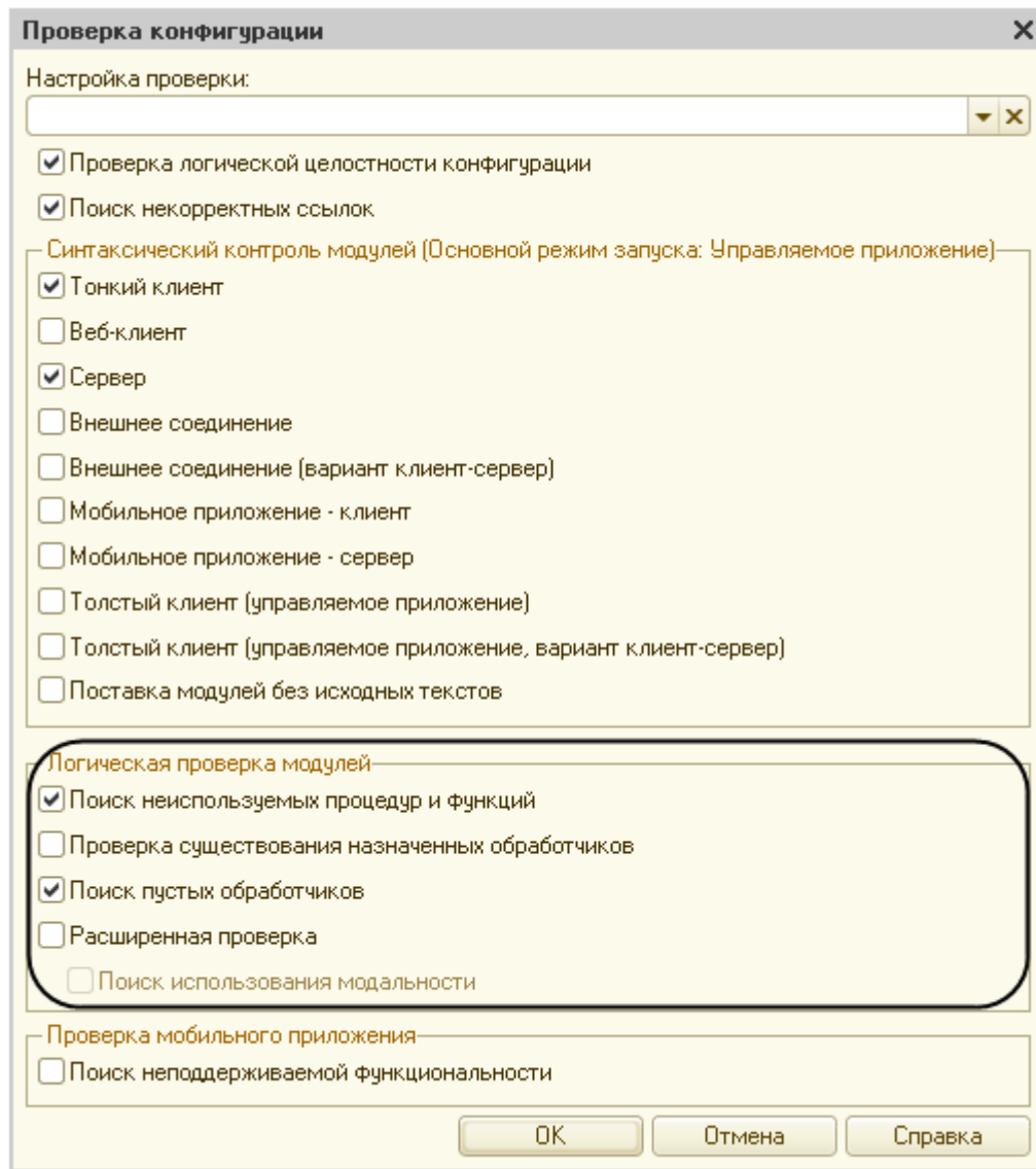
Рис. 188. Параметры проверки конфигурации
