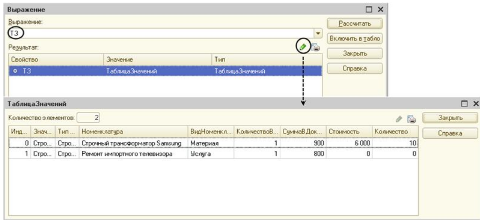
Рис. 167. Просмотр таблицы значений, содержащей результат запроса
