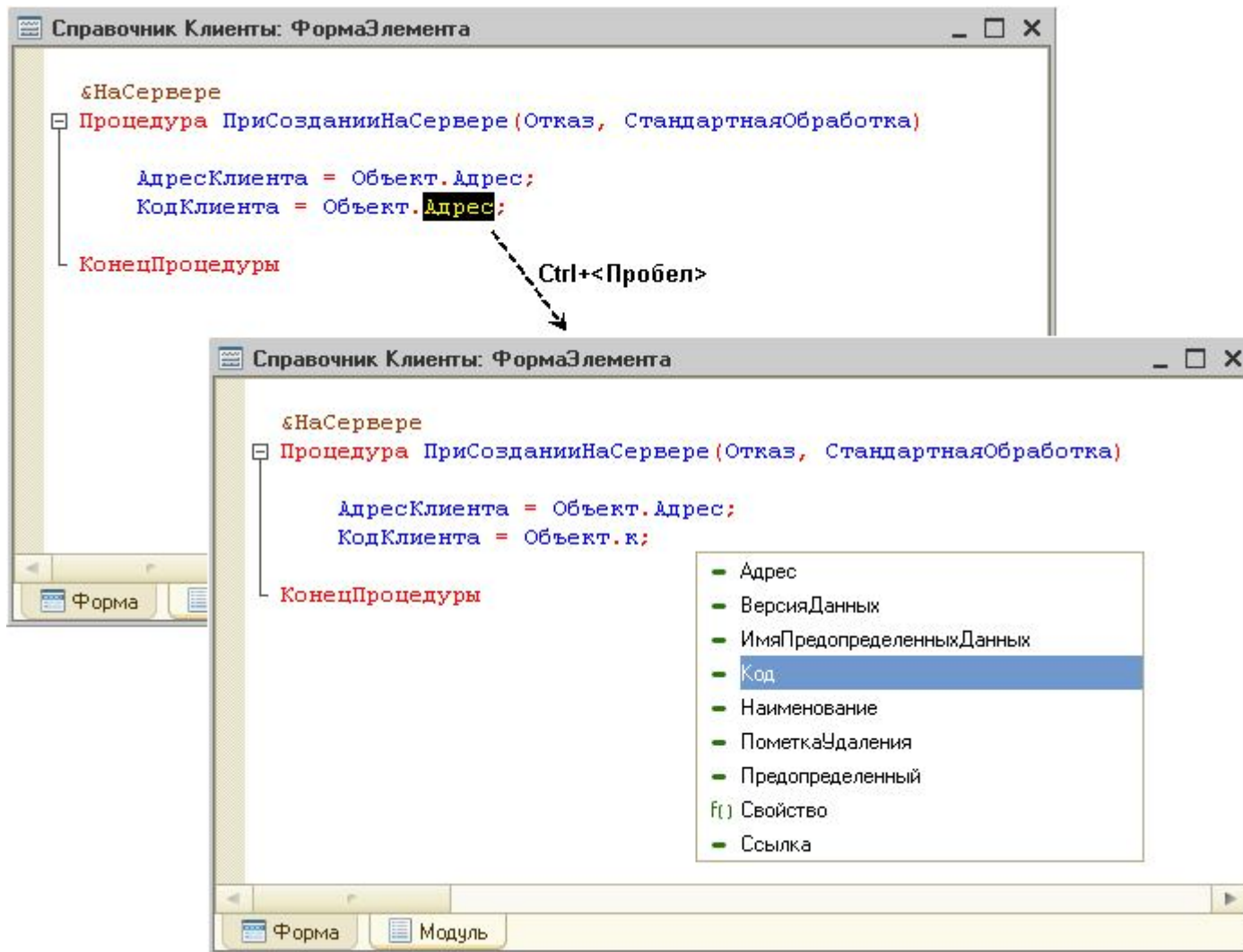
Рис. 116. Использование контекстной подсказки при изменении имени реквизита объекта
