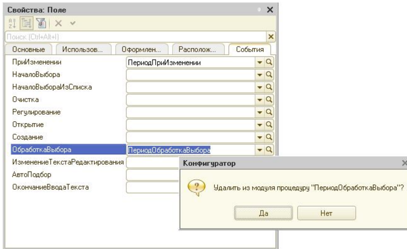
Рис. 104. Установка и удаление обработчика события
