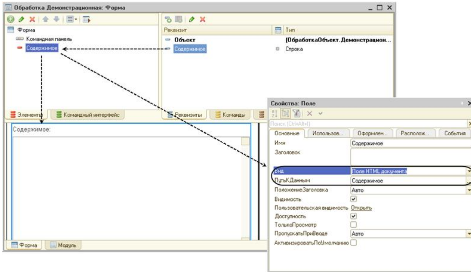
Рис. 93. Создание реквизита формы и связанного с ним поля HTML-документа
