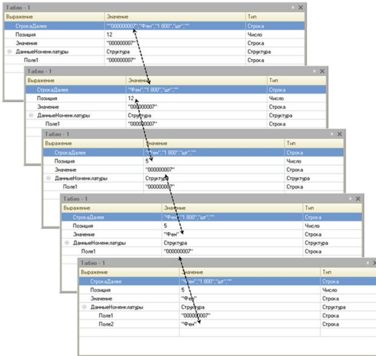
Рис. 164. Пошаговое выполнение отладки
