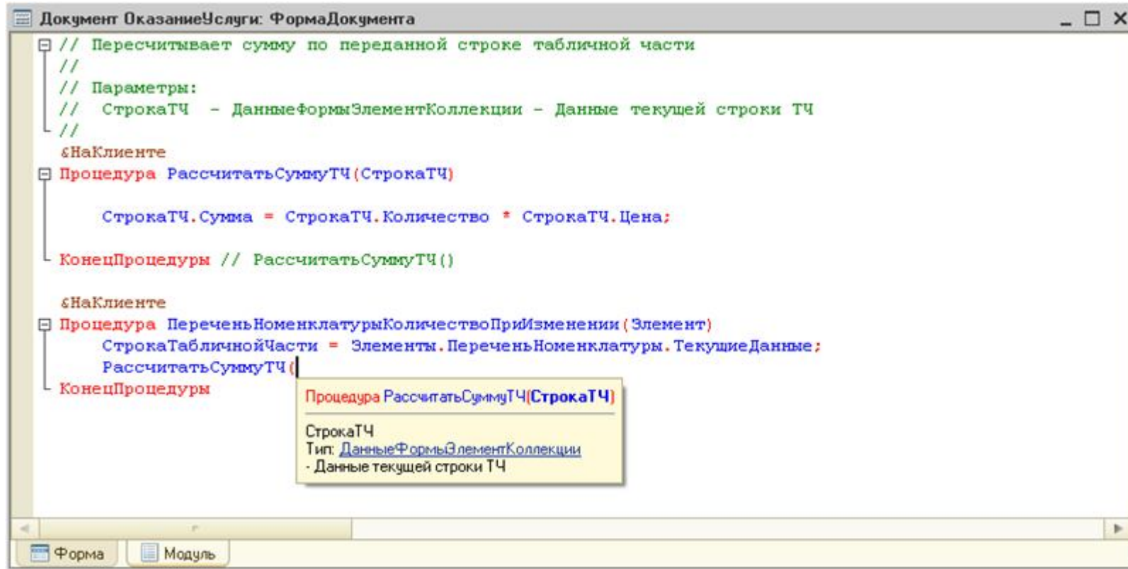
Рис. 124. Контекстная подсказка параметров созданной процедуры
