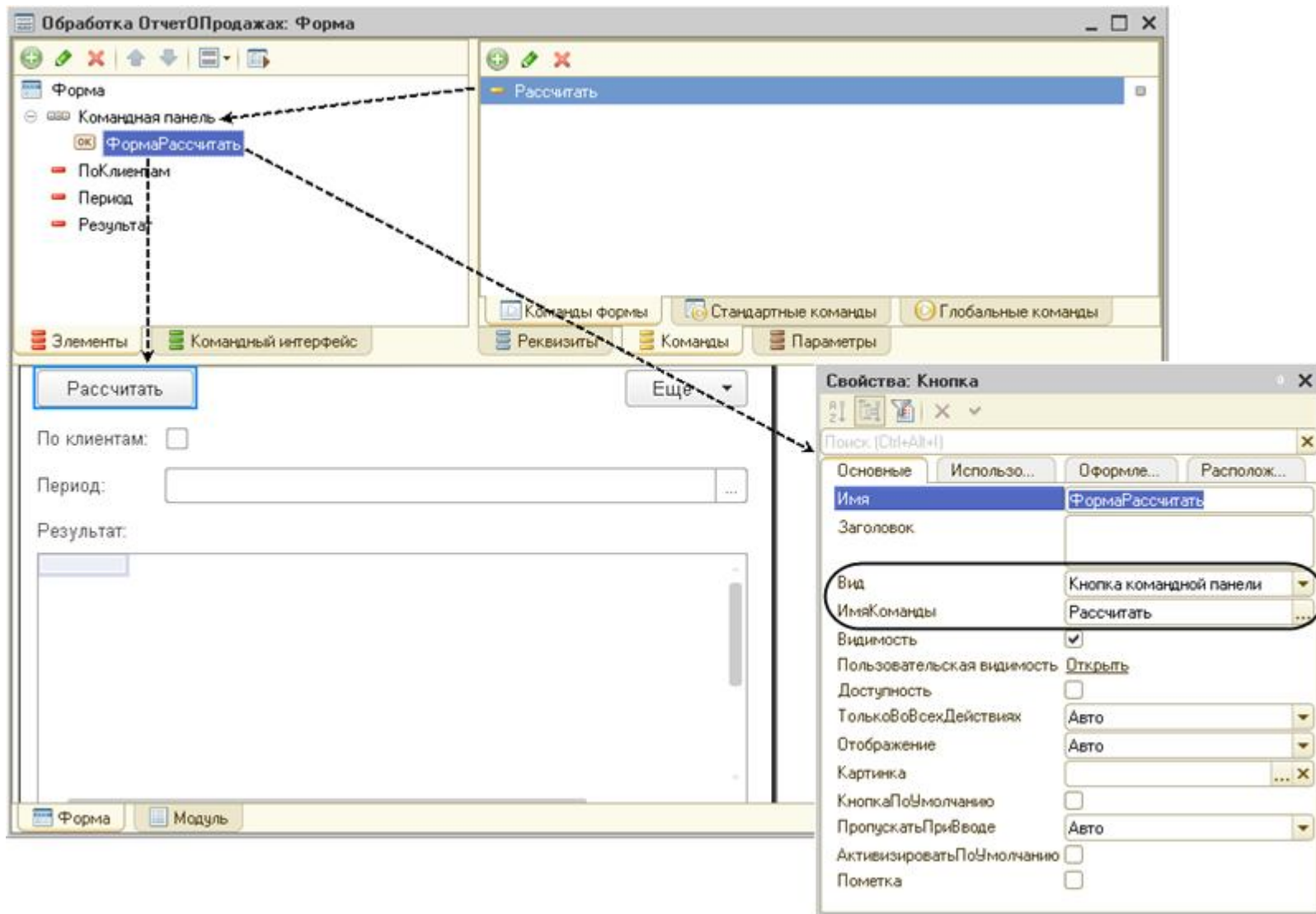
Рис. 95. Конструирование произвольной формы в редакторе формы
