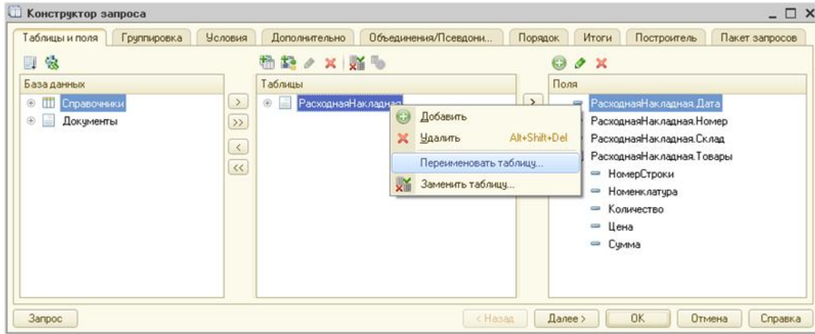
Рис. 144. Изменение псевдонима таблицы-источника в конструкторе запроса
