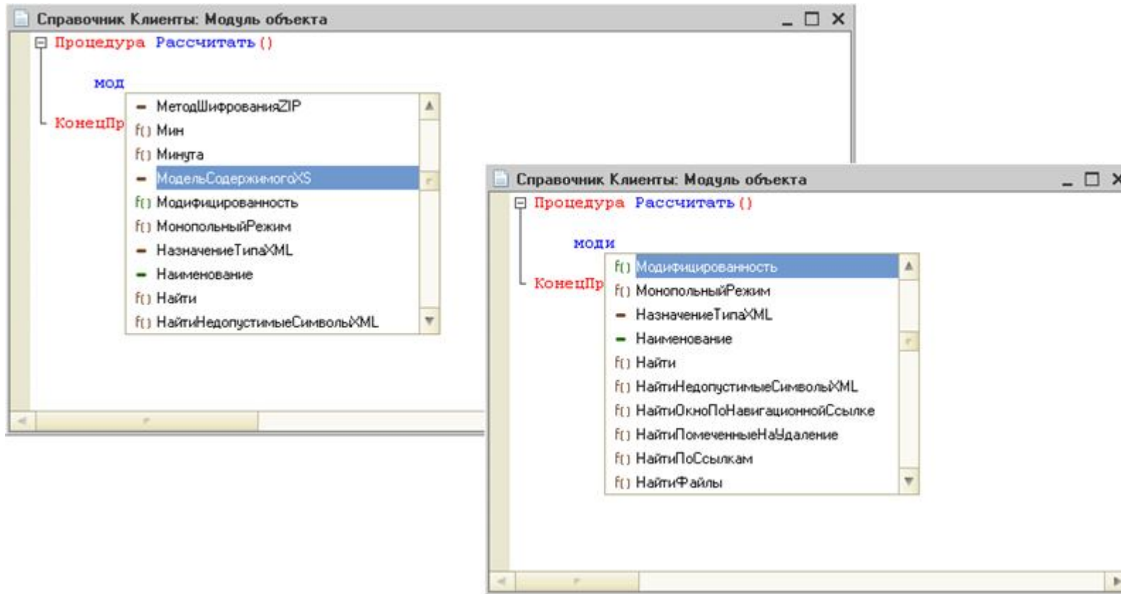
Рис. 112. Использование контекстной подсказки при написании имени метода объекта
