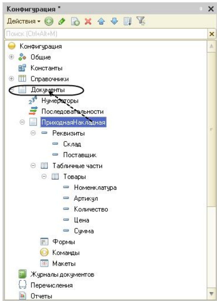
Рис. 71. Копирование объекта в дереве объектов конфигурации
