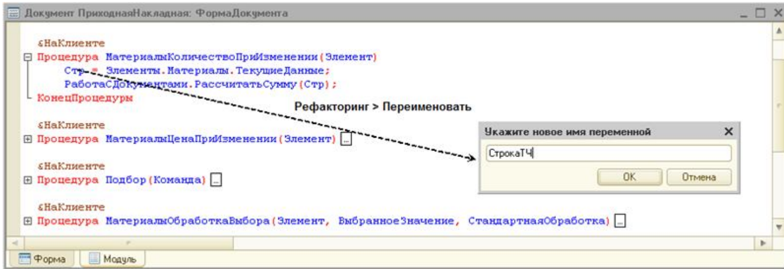
Рис. 170. Переименование локальной переменной модуля формы
