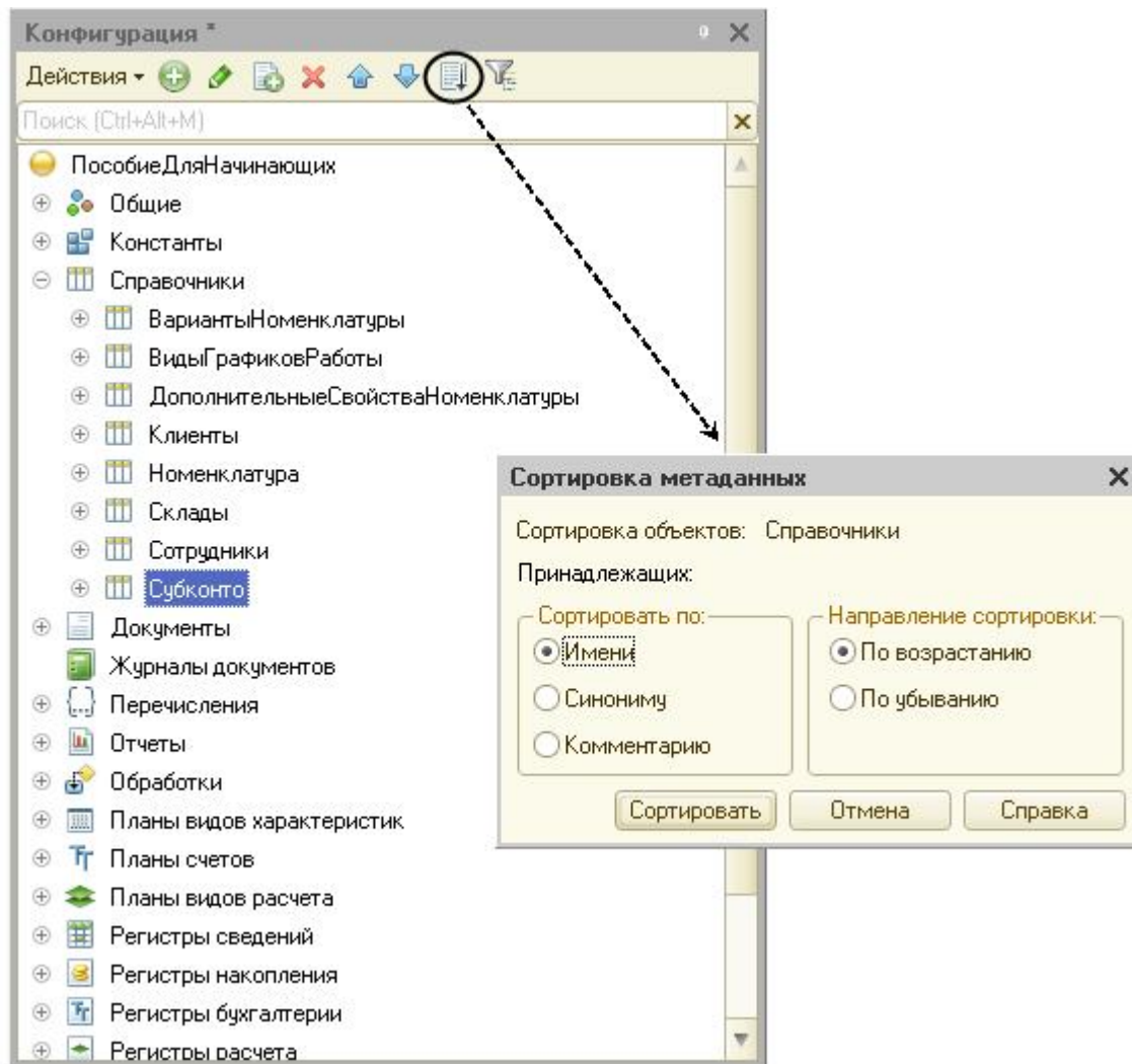
Рис. 42. Сортировка объектов в дереве объектов конфигурации
