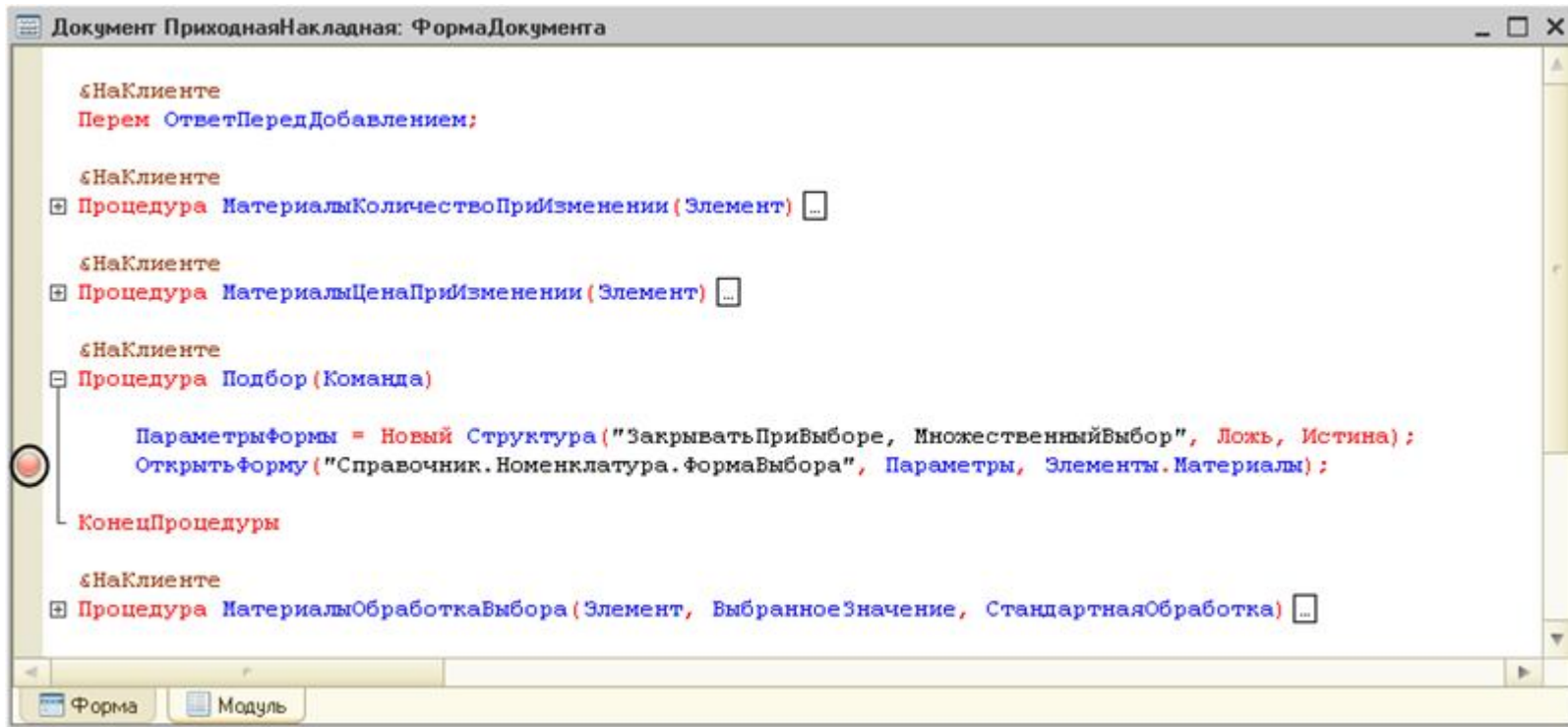
Рис. 153. Установка точки останова в тексте модуля
