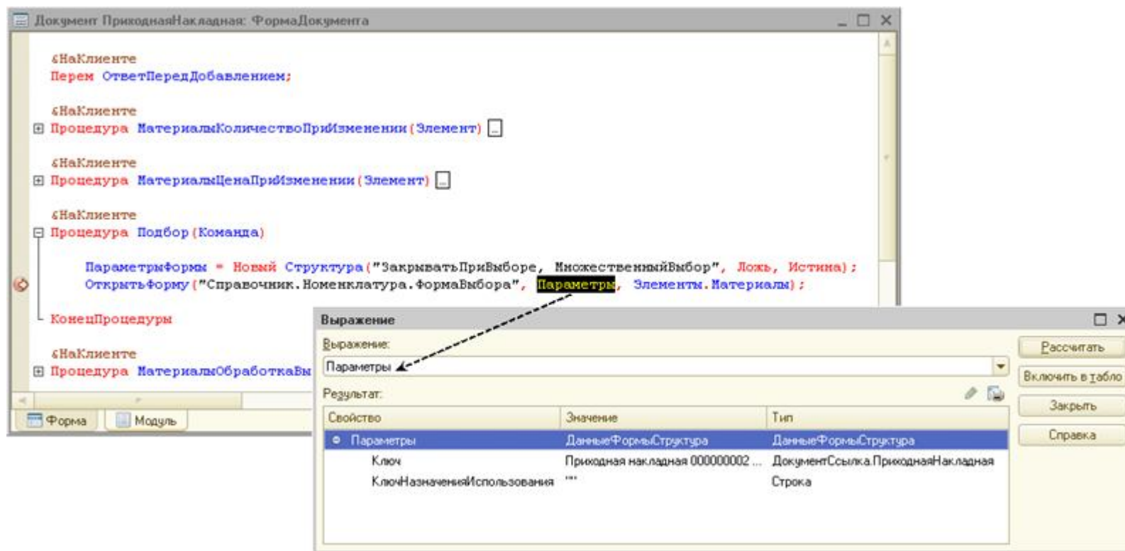
Рис. 154. Просмотр значения параметра в окне «Выражение»
