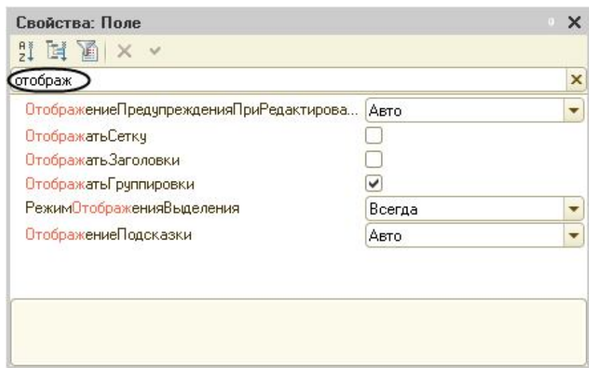
Рис. 44. Поиск свойств в строке поиска палитры свойств
