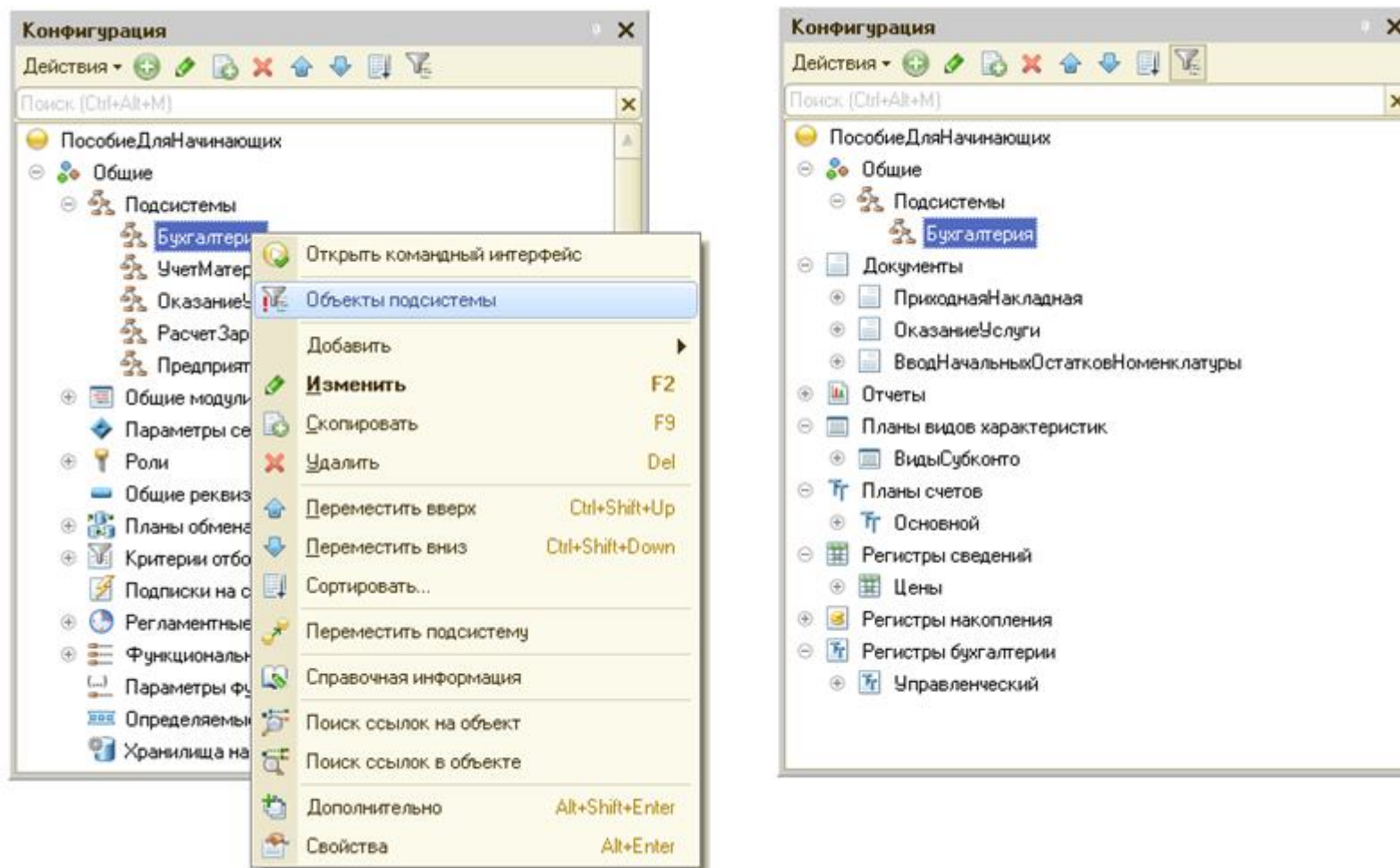
Рис. 14. Отбор объектов в дереве конфигурации по принадлежности к текущей подсистеме
