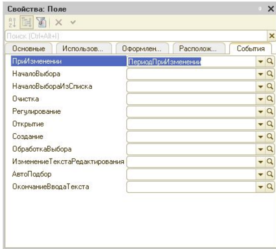
Рис. 102. Установка обработчика события
