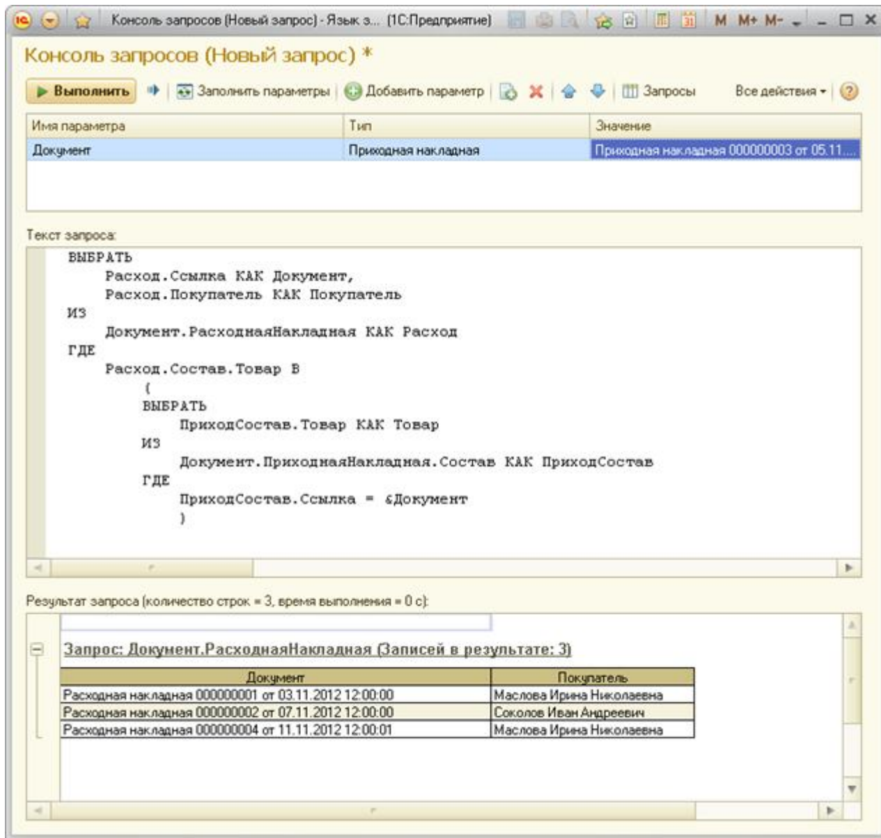
Рис. 145. Выполнение запроса в консоли запросов
