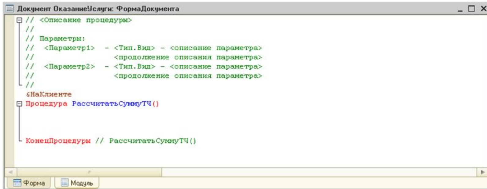
Рис. 123. Текст шаблона процедуры в модуле формы
