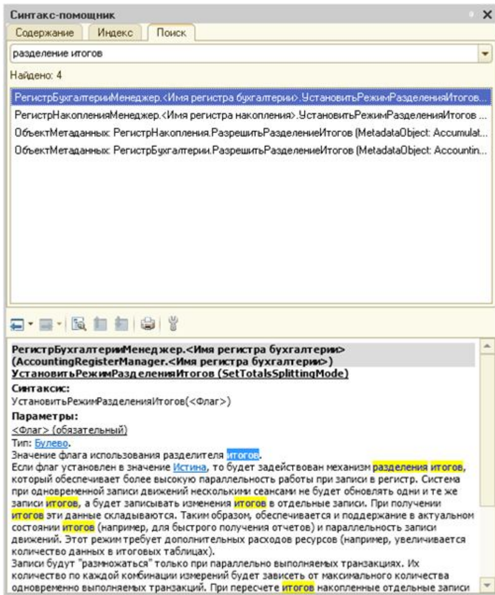
Рис. 34. Поиск по синтакс-помощнику на закладке «Поиск»
