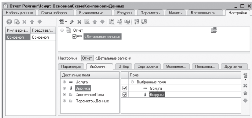
Рис. 13.35. Структура отчета «РейтингУслуг»
