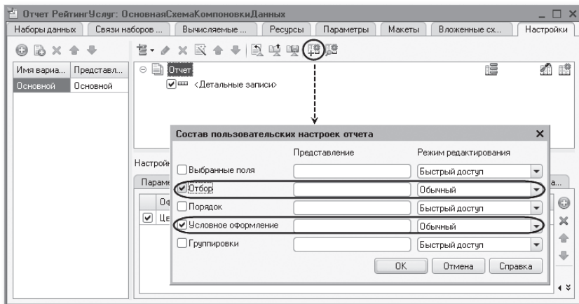
Рис. 13.49. Состав пользовательских настроек
