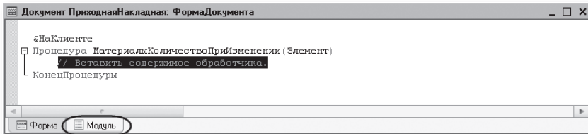
Рис. 4.23. Шаблон обработчика события «ПриИзменении» поля табличной части «Количество»
