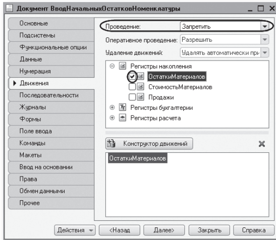
Рис. 21.1. Запрет проведения документа
