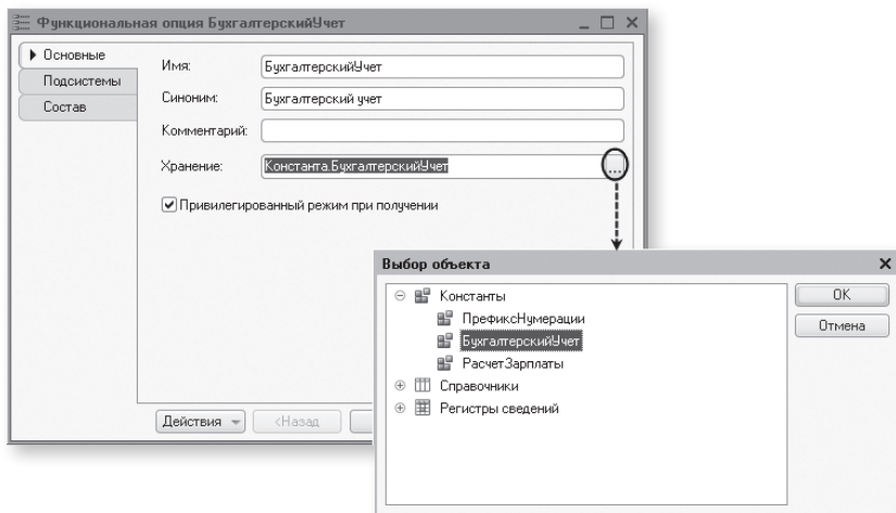
Рис. 25.2. Создание функциональной опции
