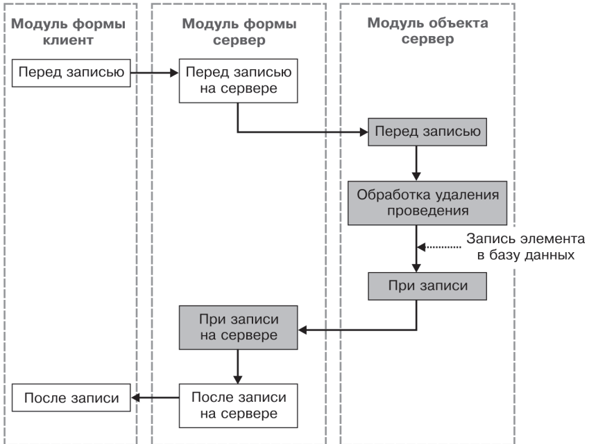
Рис. 29.8. Последовательность событий при отмене проведения документа из формы документа
