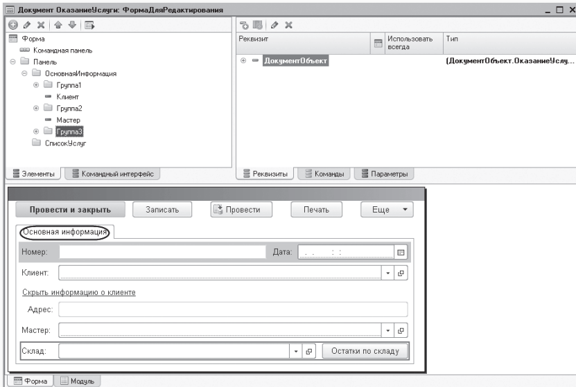
Рис. 28.23. Окно редактора формы
