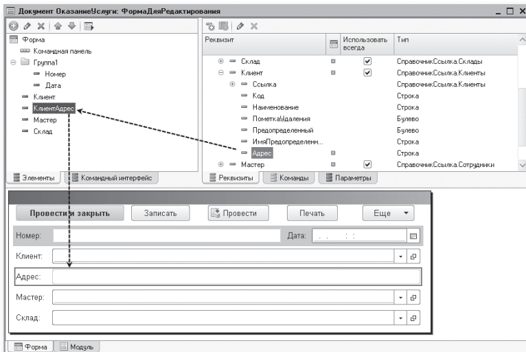
Рис. 28.15. Окно редактора формы
