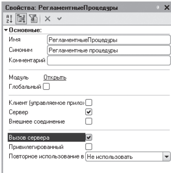
Рис. 20.2. Свойства общего модуля
