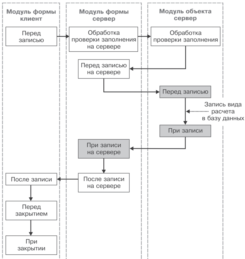
Рис. 29.15. Последовательность событий при записи вида расчета из формы вида расчета
