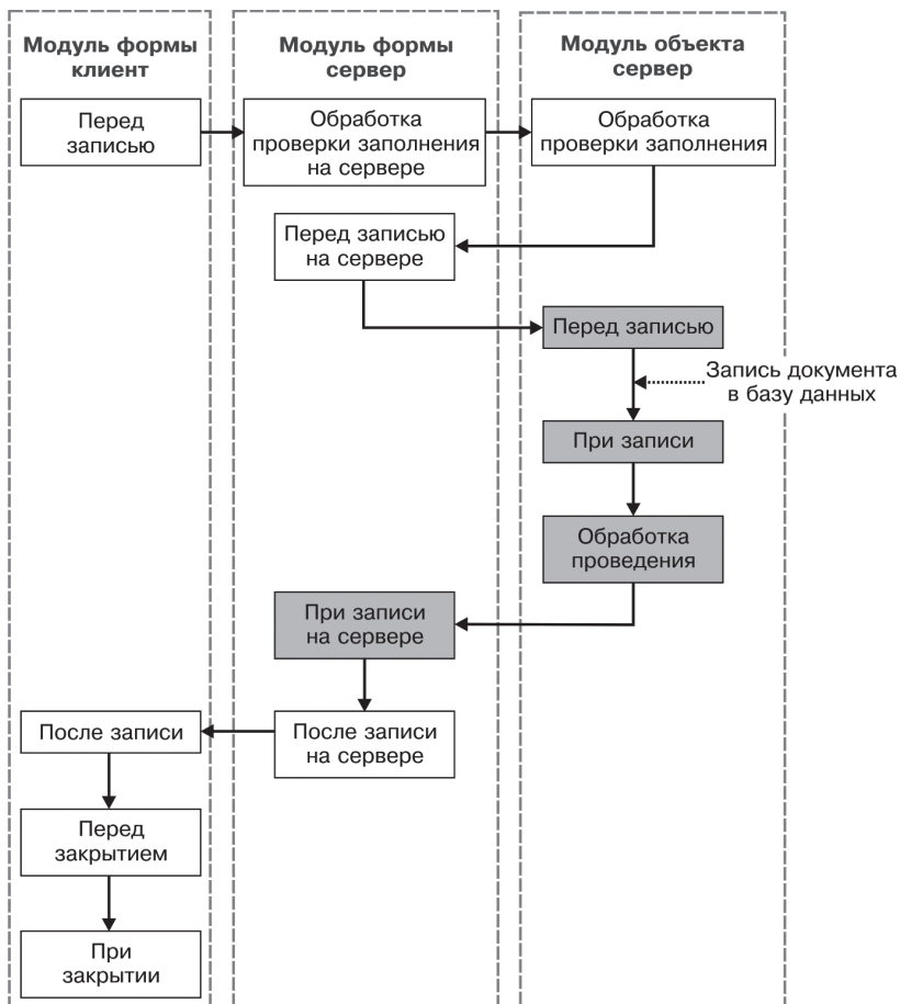
Рис. 29.7. Последовательность событий при проведении документа из формы документа
