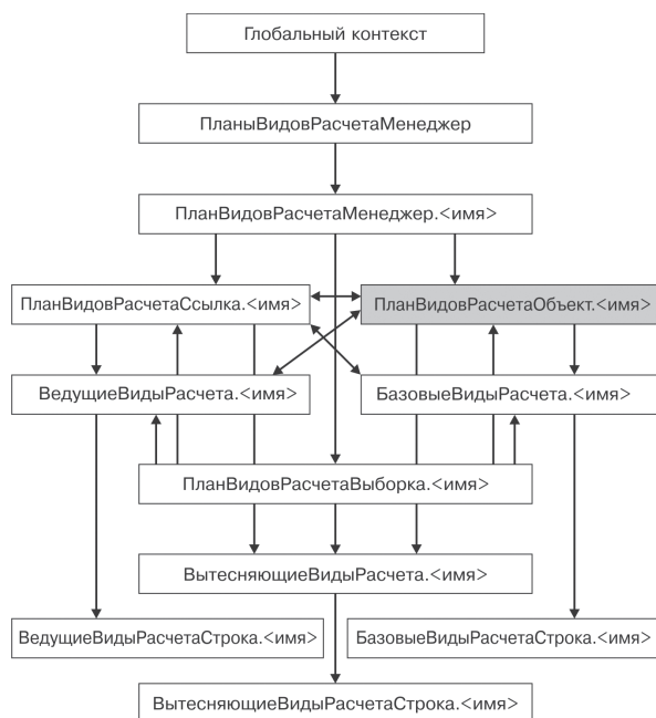
Рис. 29.14. Объекты встроенного языка для работы с планами видов расчета
