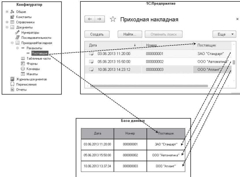
Рис. 4.2. Реквизит «Поставщик» документа «Приходная накладная» в режиме «Конфигуратор», в режиме «1С:Предприятие» и в базе данных
