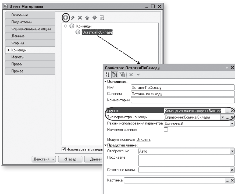
Рис. 27.37. Создание параметризованной команды
