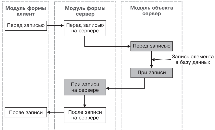
Рис. 29.6. Последовательность событий при записи нового документа из формы документа
