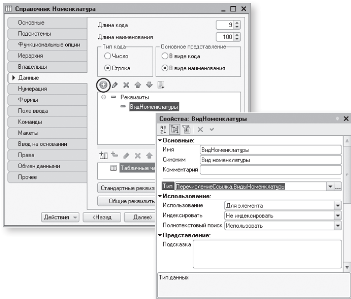
Рис. 10.2. Данные справочника «Номенклатура»
