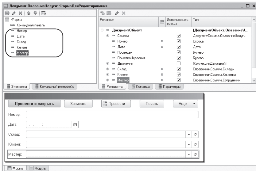
Рис. 28.11. Окно редактора формы
