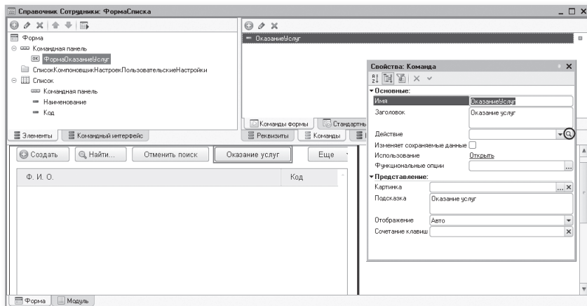
Рис. 27.40. Форма списка справочника «Сотрудники»
