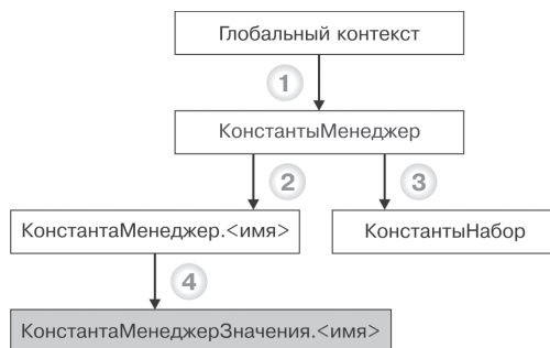
Рис. 29.1. Объекты встроенного языка для работы с константами
