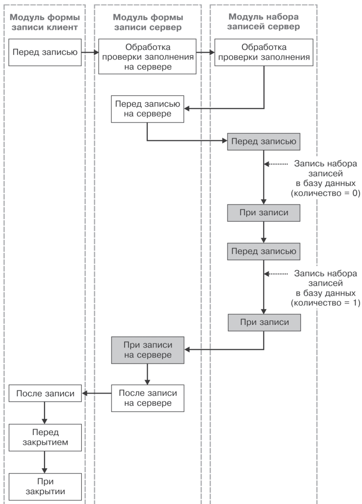
Рис. 29.17. Последовательность событий при сохранении данных из формы записи регистра сведений
