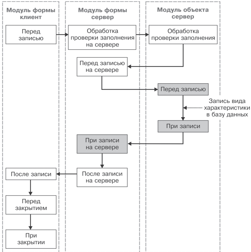
Рис. 29.11. Последовательность событий при записи вида характеристики из формы элемента
