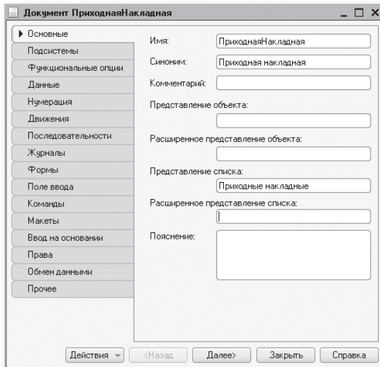
Рис. 4.4. Установка основных свойств документа
