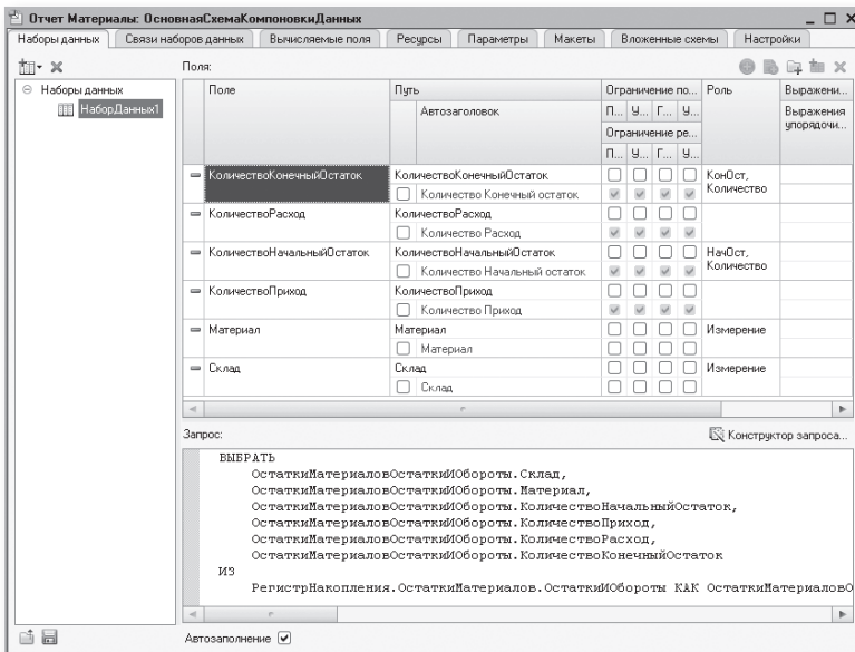
Рис. 7.10. Конструктор схемы компоновки данных
