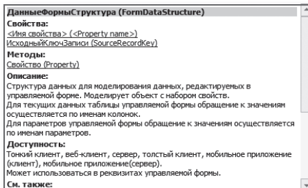
Рис. 5.31. Описание объекта «ДанныеФормыСтруктура» в синтакс-помощнике
