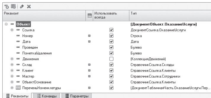
Рис. 28.4. Закладка «Реквизиты» редактора формы
