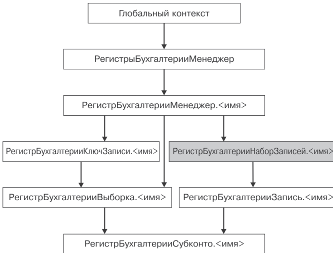
Рис. 29.21. Объекты встроенного языка для работы с регистрами бухгалтерии
