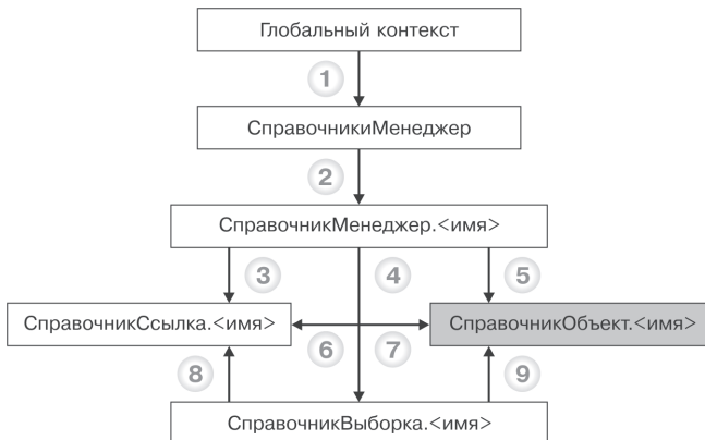
Рис. 29.3. Объекты встроенного языка для работы со справочниками
