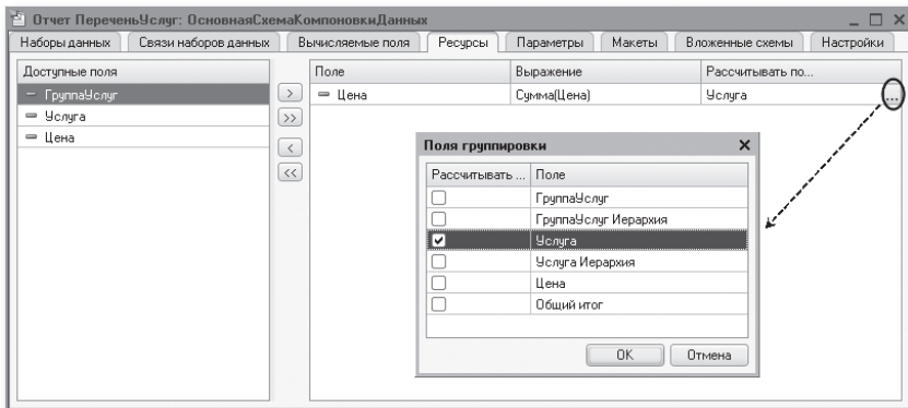
Рис. 13.91. Ресурсы схемы компоновки
