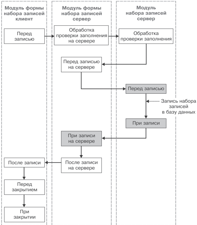
Рис. 29.22. Последовательность событий при сохранении набора записей регистра бухгалтерии из формы
