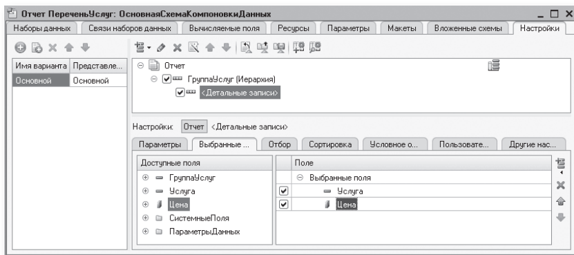
Рис. 13.94. Структура и поля отчета
