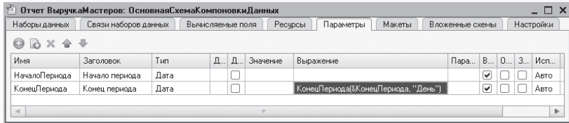
Рис. 13.62. Параметры компоновки данных
