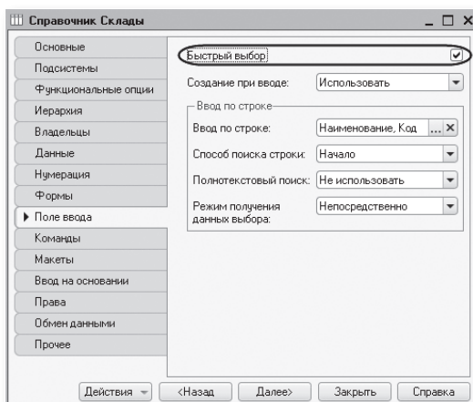
Рис. 3.67. Установка свойства «Быстрый выбор»
