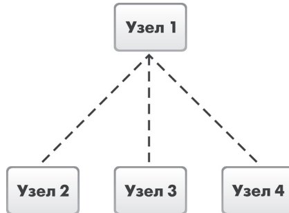
Рис. 24.35. Информационная база из отдельных информационных баз с идентичной конфигурацией
