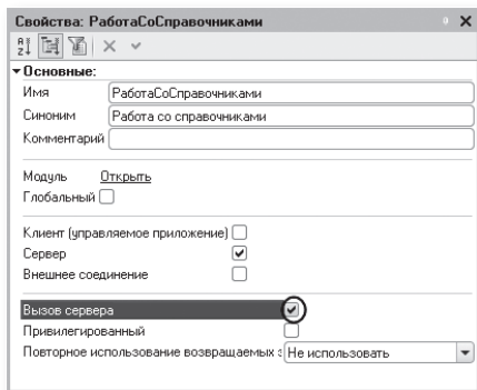
Рис. 9.9. Свойства общего модуля
