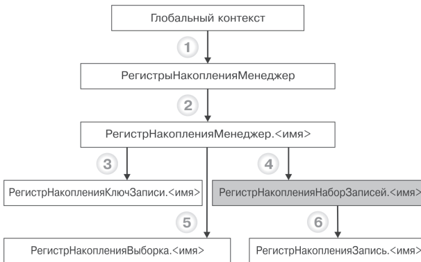
Рис. 29.19. Объекты встроенного языка для работы с регистрами накопления
