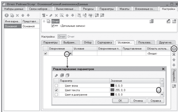
Рис. 13.43. Настройка условного оформления
