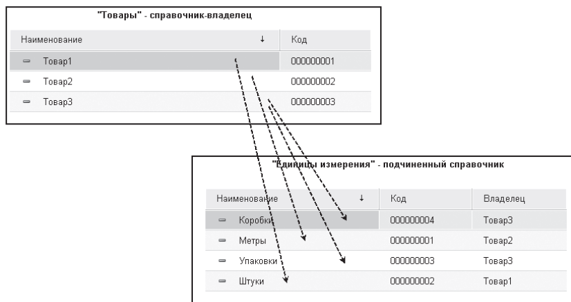
Рис. 3.7. Справочник «Товары» – владелец справочника «Единицы измерения»
