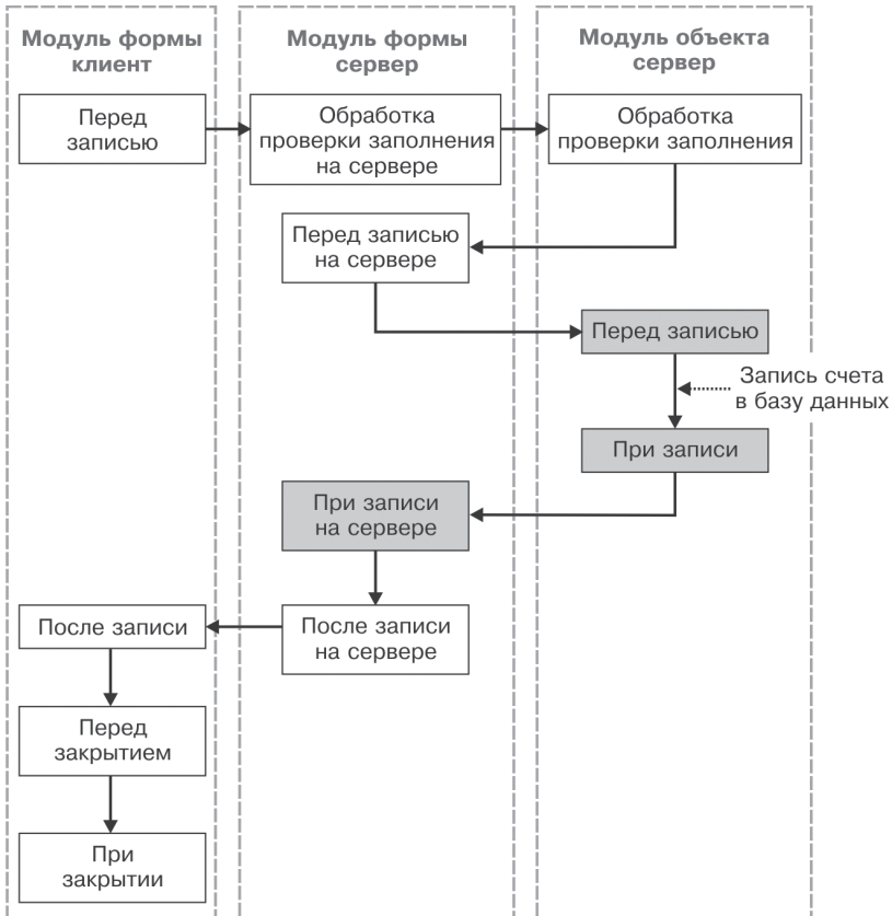
Рис. 29.13. Последовательность событий при записи счета из формы счета
