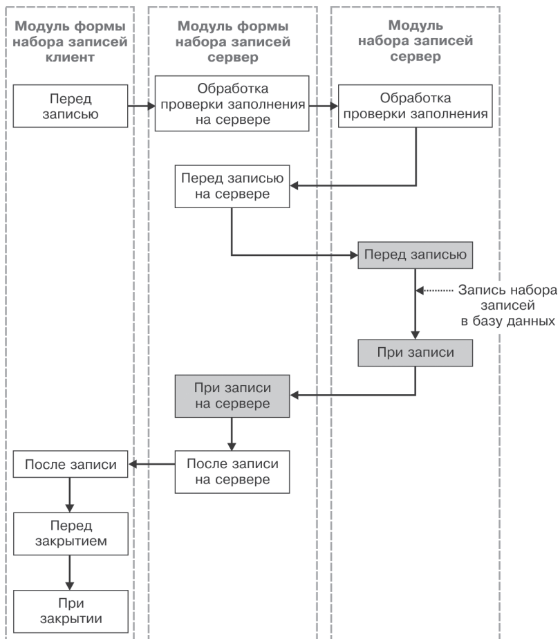
Рис. 29.20. Последовательность событий при сохранении набора записей регистра накопления из формы набора записей
