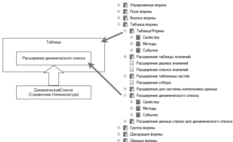
Рис. 27.5. Контекст таблицы дополняется контекстом расширения динамического списка
