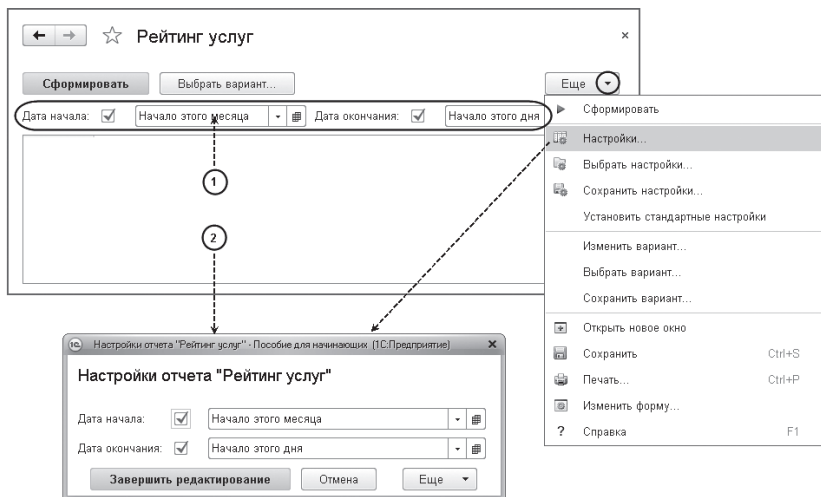
Рис. 13.38. Быстрые (1) и обычные (2) пользовательские настройки
