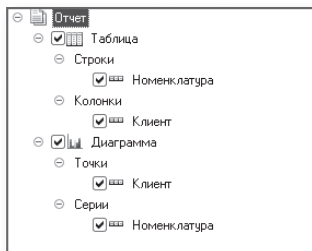
Рис. 13.4. Возможная структура отчета
