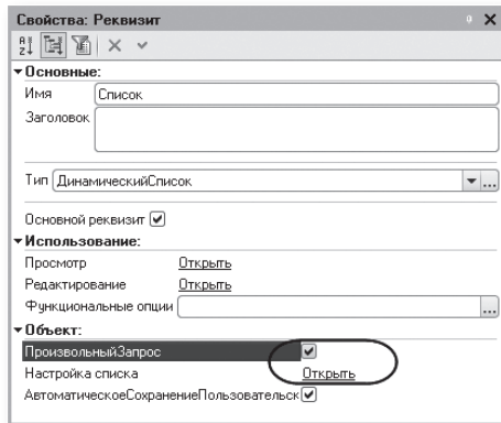
Рис. 27.16. Вызов настройки динамического списка
