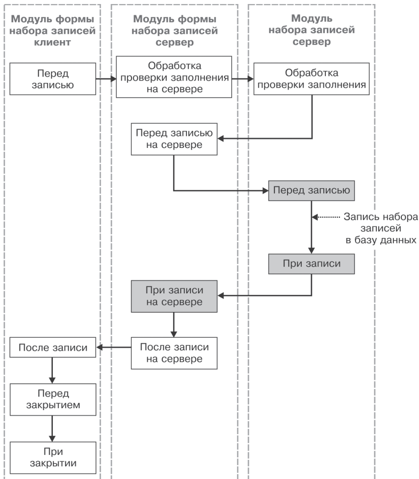
Рис. 29.24. Последовательность событий при сохранении набора записей регистра расчета из формы
