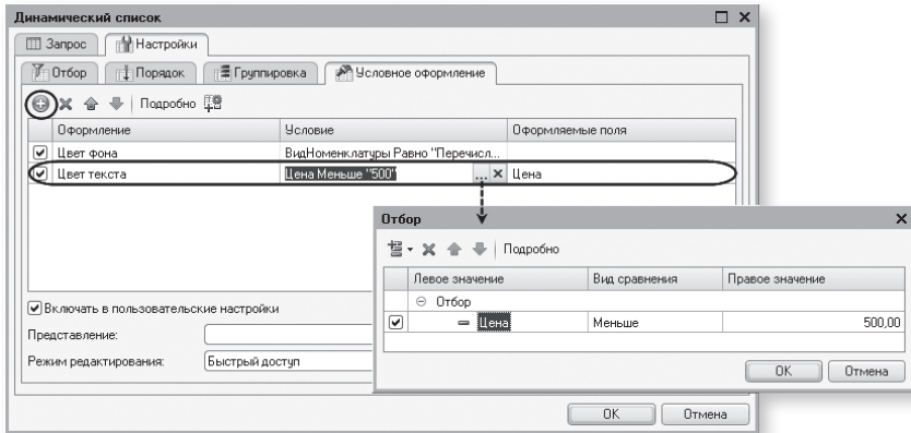
Рис. 27.20. Настройка условного оформления динамического списка
