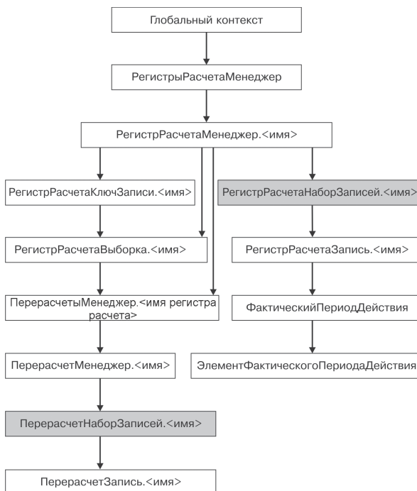
Рис. 29.23. Объекты встроенного языка для работы с регистрами расчетов
